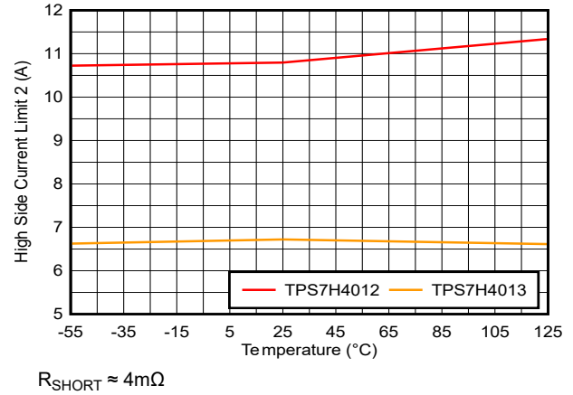
図 7-38. ハイサイド電流制限スレッシュホールド 2 (I OC_HS2 ) と温度との関係
