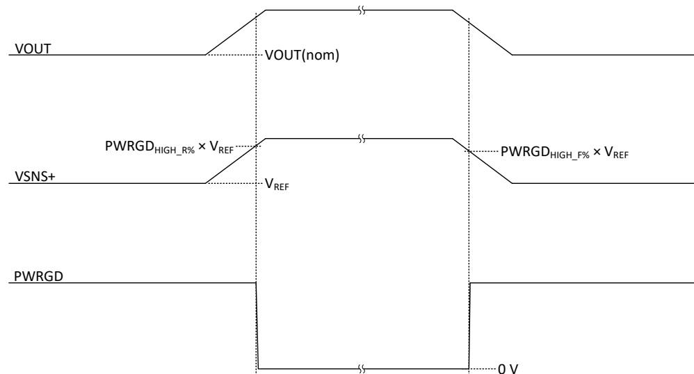
図 9-3. パワーグッドの HIGH スレッシュホルド
