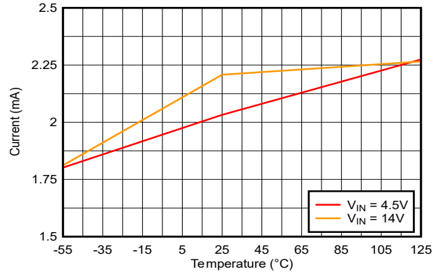
図 7-26. V_{IN} シャットダウン電流と温度との関係
