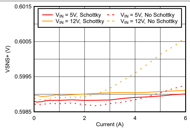
図 7-32. 1MHz での VSNS+ と出力電流の関係
