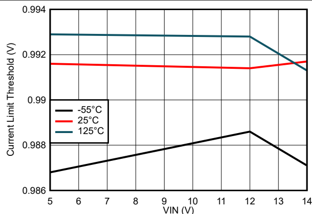
図 6-23. 電流制限スレッシュホールドと入力電圧との関係
