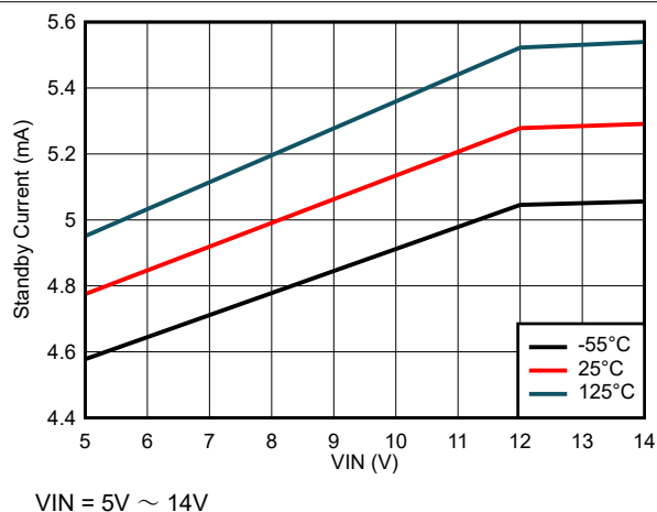
図 6-33. スタンバイ電流と入力電圧との関係
