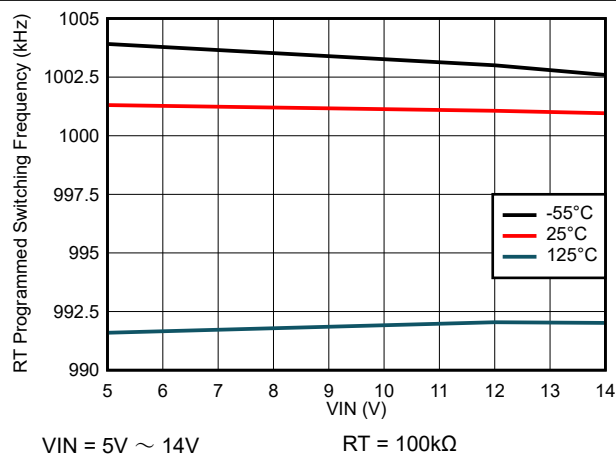
図 6-19. スwitchング周波数と入力電圧との関係
