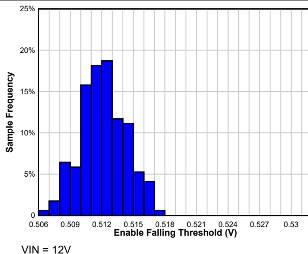
図 6-44. T_A = -55^\circ\text{C} での立ち下がりスレッシュホールド分布をイネーブル
