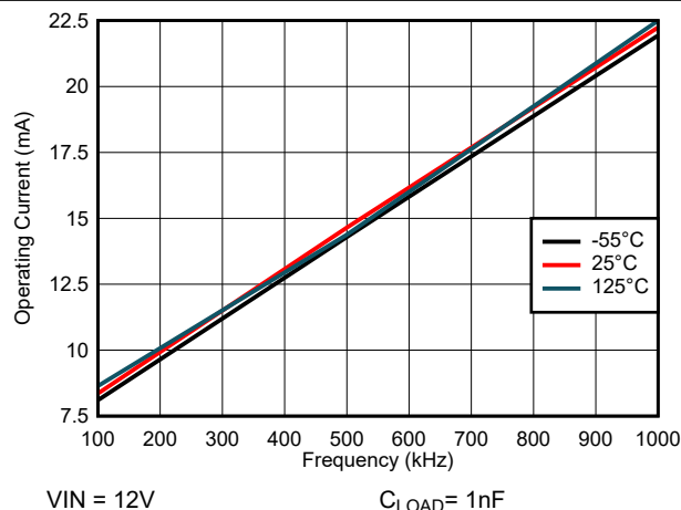
図 6-31. 動作供給電流と周波数との関係
