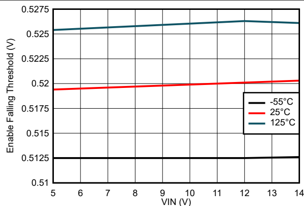
図 6-11. イネーブル立ち下がりスレッシュホールドと入力電圧との関係
