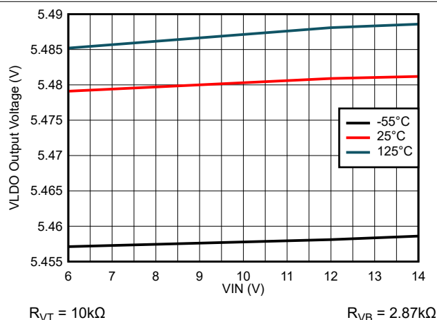
図 6-3. 内部リニア レギュレータの出力電圧と入力電圧との関係
