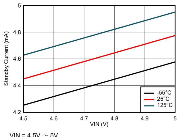
図 6-32. スタンバイ電流と入力電圧との関係
