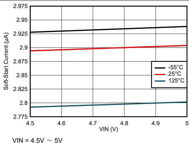
図 6-34. ソフトスタート電流と入力電圧との関係
