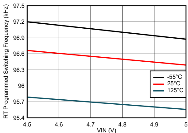
図 6-12. スイッチング周波数と入力電圧との関係
