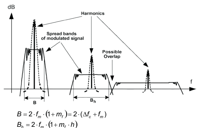
図 46. 方形波信号により変調された高調波の拡散帯域幅
