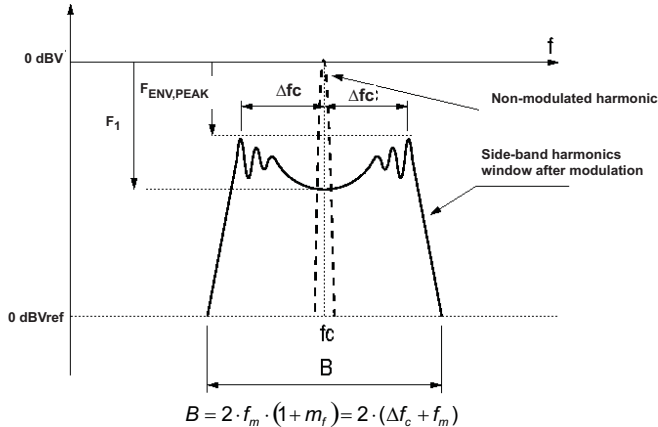
図 45. 正弦波状に時間軸で周波数変調された正弦波のスペクトラム。
