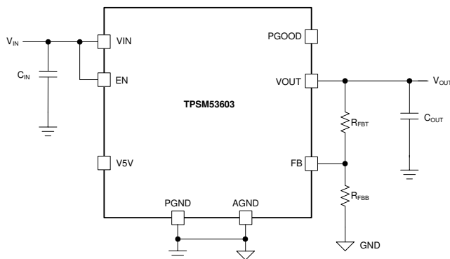
概略回路図
