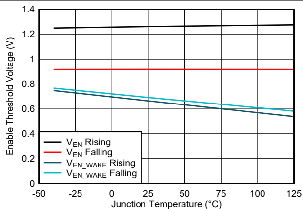
図 7-6. Enable Thresholds
