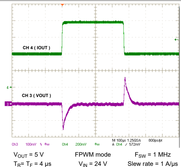
図 9-7. Load Transient, 4 A to 8 A, 1 A/ \mu\text{s}
