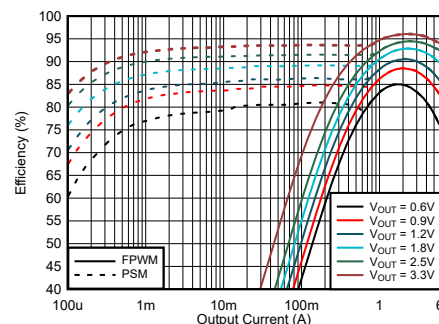
TPSM8286AA0HRDMR – 効率と出力電流との関係、 V IN = 5.0V
