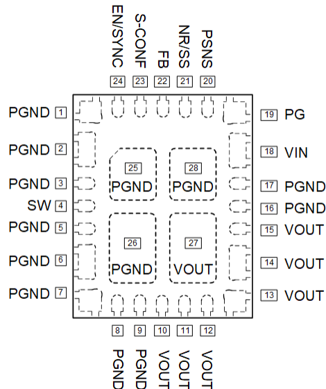
図 5-1. 28-Pin QFN RDU Package (Top View)
