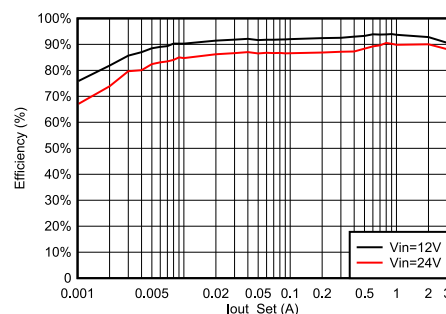
TPSM84338 の効率 ( V_{OUT} = 5V 、 f_{sw} = 1000kHz )
