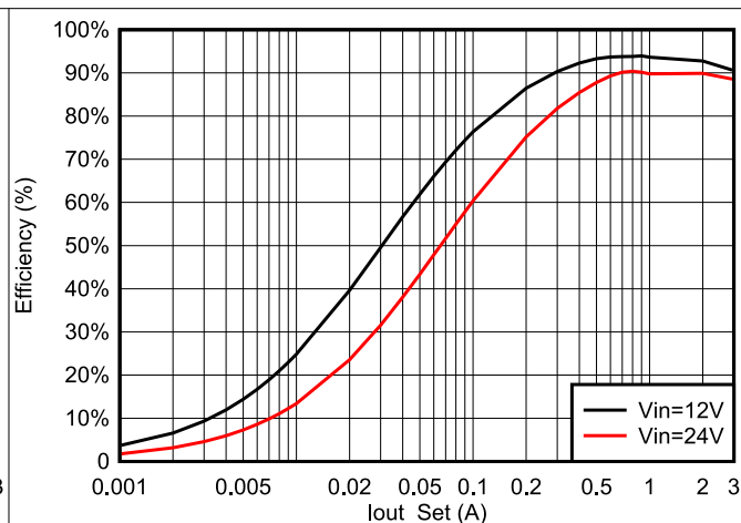
図 7-3. Efficiency (FCCM)
