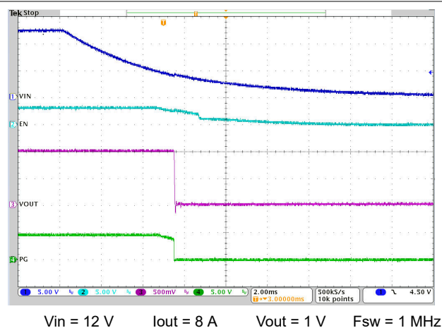
図 8-14. VIN Shutdown
