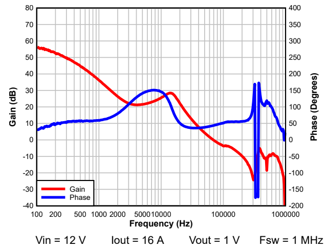
图 8-7. Bode Plot
