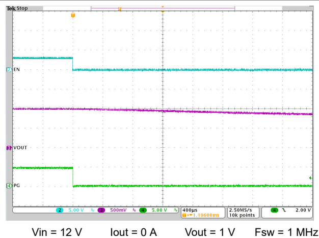
図 8-10. EN Shutdown
