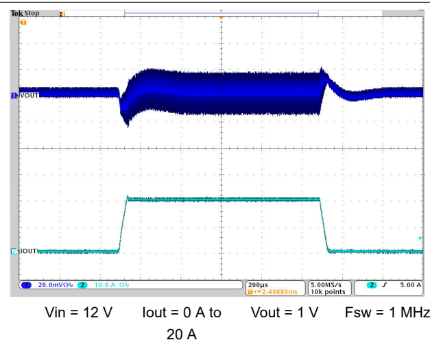
图 8-8. Load Transient
