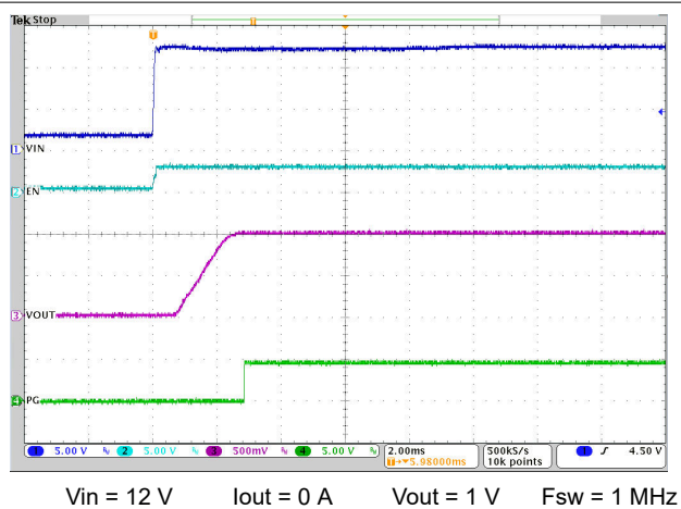
図 8-13. VIN Start-Up
