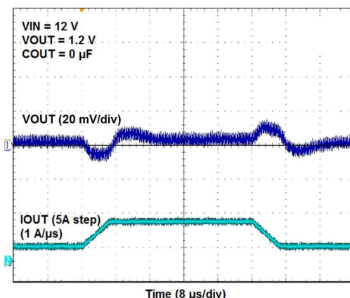
過渡応答
