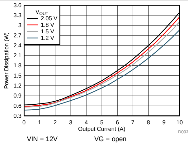
图 3. Power Dissipation
