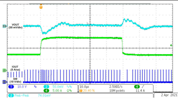
I_{STEP} = 7.5\text{ A} - 15\text{ A} - 7.5\text{ A} 5 A/μs 8-37. Transient Response, V_{PP} = 74\text{ mV}
