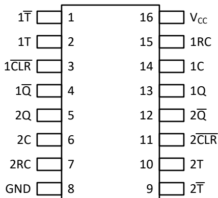
図 4-1. TPUL2G122 D および PW パッケージ 16 ピン SOIC および TSSOP 上面図
