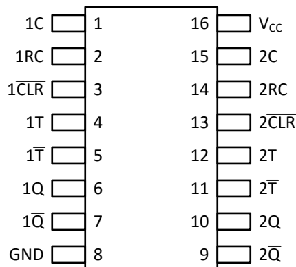
図 4-2. TPUL2G122A D および PW パッケージ 16 ピン SOIC および TSSOP 上面図
