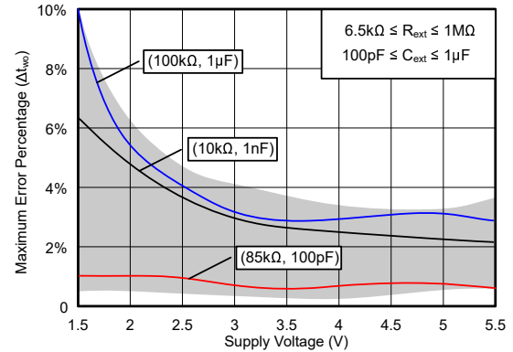
図 5-23. 電源電圧における最大出力パルス幅誤差 (絶対値)
