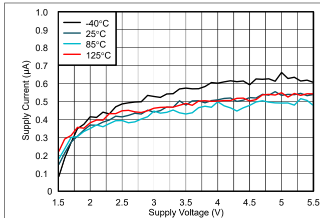
図 5-2. 電源電流と電源電圧との関係
