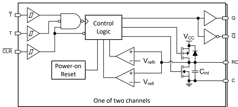
図 7-4. TPUL2T122A
