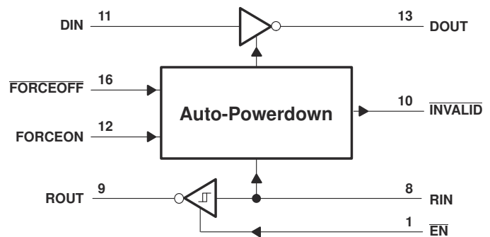
概略回路図
