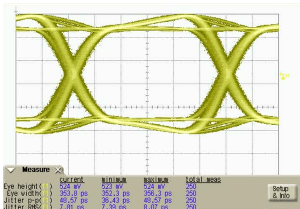
图 11-2. TSB82AF15-EP Eye Diagram
