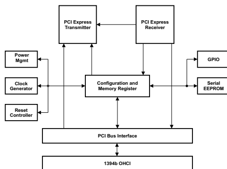
概要ブロック図
