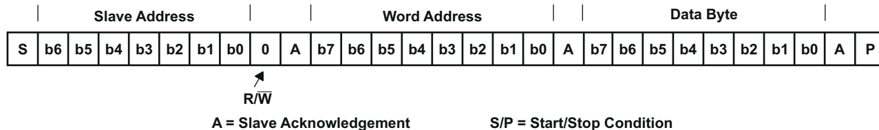
10-9. Serial-Bus Protocol Byte Write
