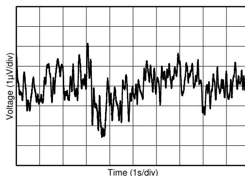
図 7-14. 0.1Hz~10Hz の入力電圧ノイズ
