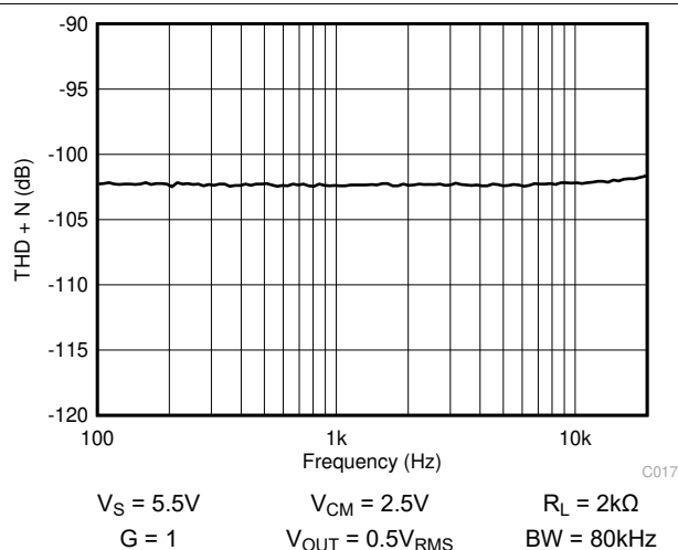
図 7-16. THD + N と周波数との関係
