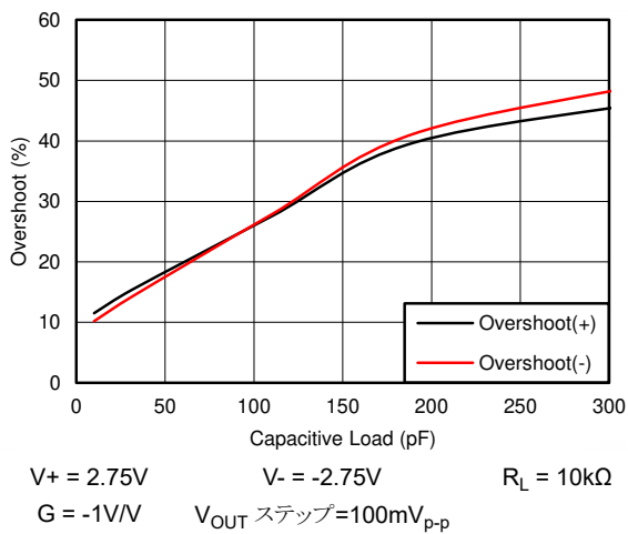
図 7-23. 小信号のオーバーシュートと負荷容量との関係
