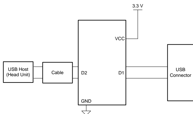
概略回路図
