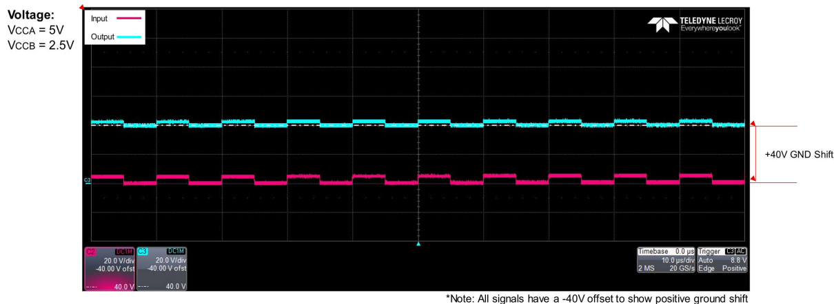
図 8-2. 5V から 2.5V への I/O 変換による -40V (上) および +40V (下) のグラウンド シフトを示す波形
