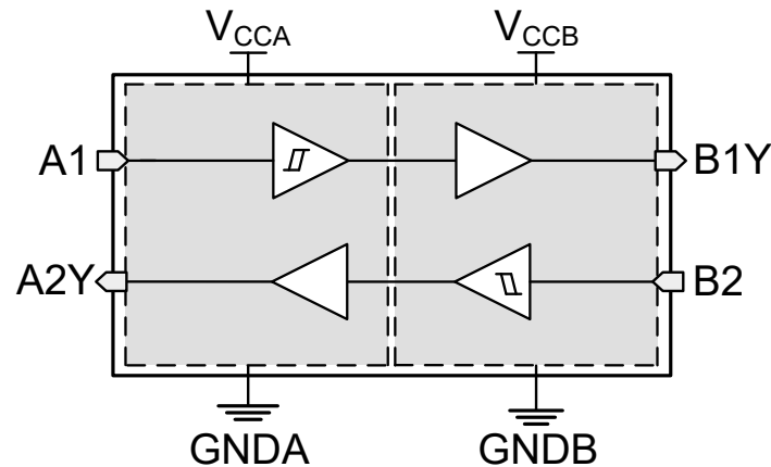
図 7-1. TXG4021 機能ブロック図
