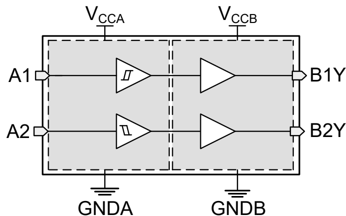
図 7-2. TXG4020 機能ブロック図
