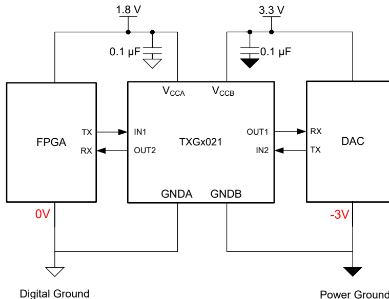
図 8-1. 試験および測定機器分野の TXG4021
