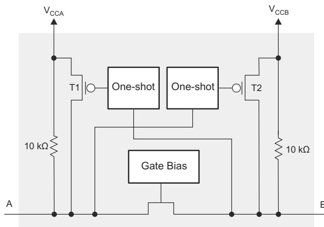
図 7-1. TXS0104W セルのアーキテクチャ
