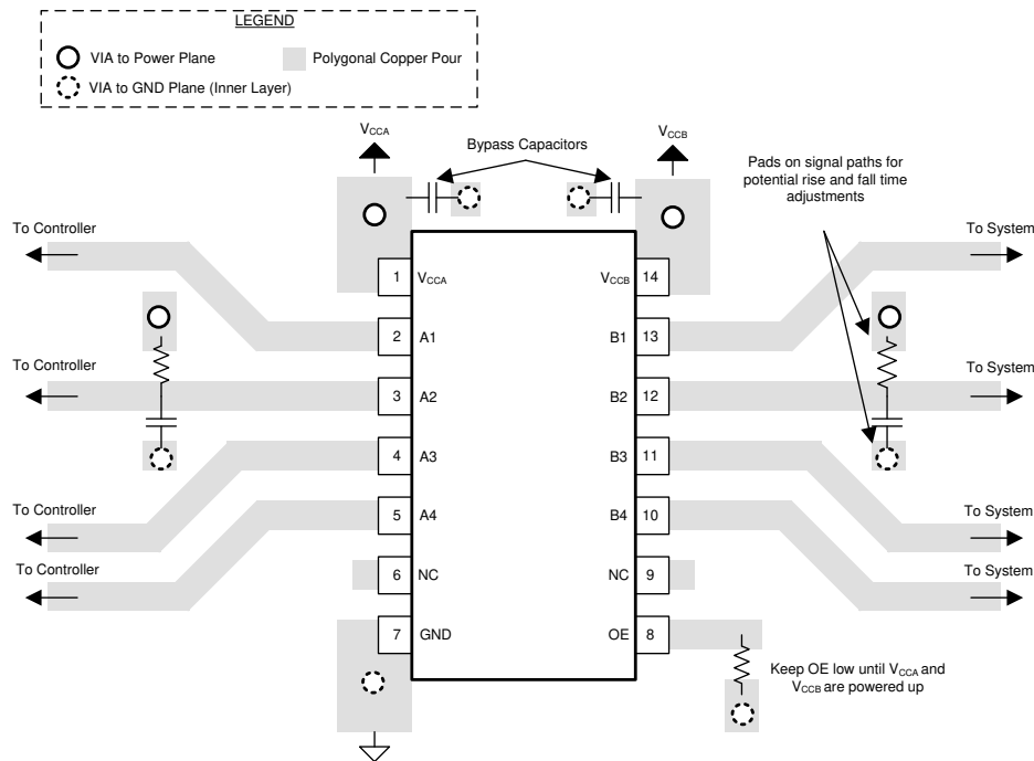
図 8-3. TXS0104W レイアウト例
