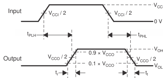
図 6-5. 伝搬遅延時間
