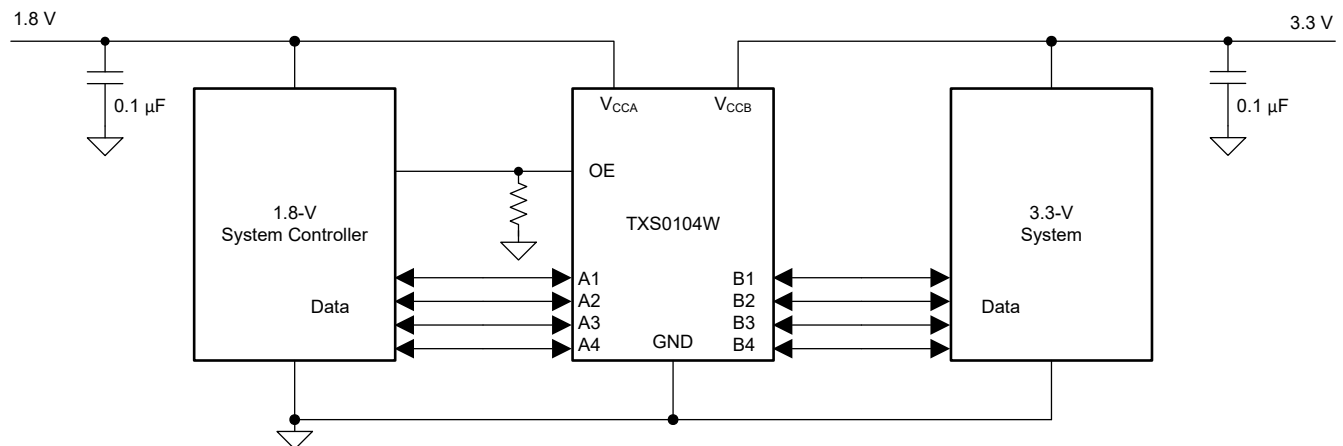
図 8-1. アプリケーション回路図
