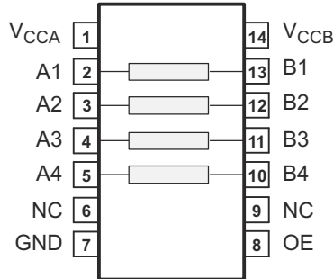
図 4-1. BQA パッケージ、14 ピン WQFN (上面図)
