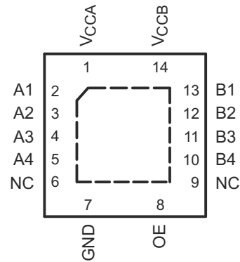
図 4-2. RGY パッケージ、14 ピン VQFN (上面図)
