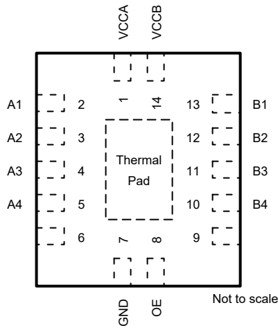
図 4-1. BQA パッケージ、14 ピン WQFN (上面図)
