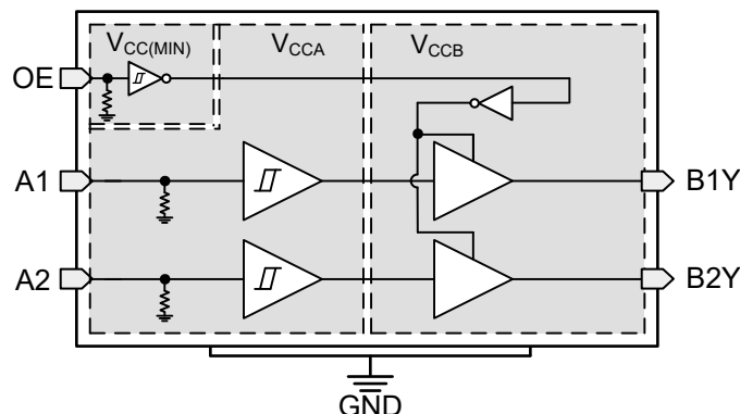
TXU0102 の機能ブロック図
