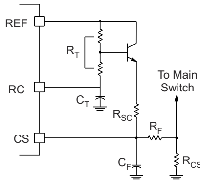
図 7-22. スローブ補償の追加
