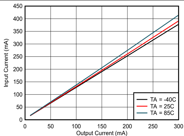
図 6-12. 入力電流 ( I_{VINP} ) と負荷電流 ( I_{VCC} ) との関係 : V_{CC} = 3.3V , V_{INP} = 5.0V , C_{OUT2} = 22\mu F
