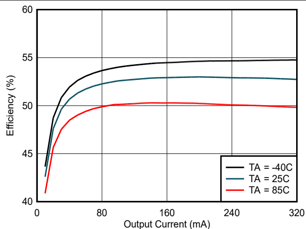
図 6-10. 効率と負荷電流 ( I_{VCC} ) との関係 : V_{CC} = 3.7V , V_{INP} = 5.0V , C_{OUT2} = 22\mu F
