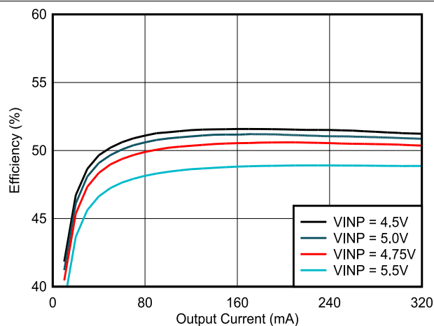
図 6-7. 効率と負荷電流 ( I_{VCC} ) との関係 : V_{CC} = 3.3V , T_A = 25^\circ C , C_{OUT2} = 22\mu F
