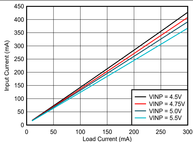
図 6-11. 入力電流 ( I_{VINP} ) と負荷電流 ( I_{VCC} ) との関係 : V_{CC} = 3.3V , T_A = 25^\circ C , C_{OUT2} = 22\mu F
