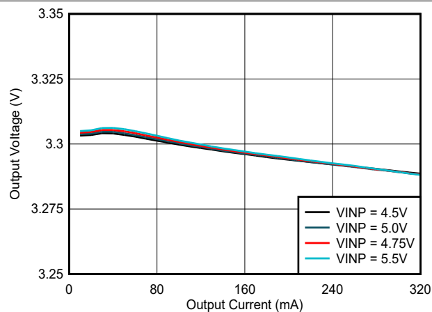
図 6-13. 出力電圧制御 ( V_{VCC} ) と負荷電流 ( I_{VCC} ) との関係 : V_{CC} = 3.3V , T_A = 25^\circ C , C_{OUT2} = 22\mu F
