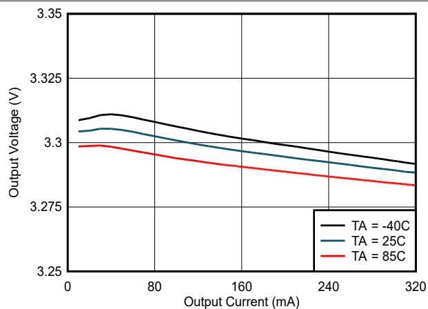
図 6-14. 出力電圧制御 ( V_{VCC} ) と負荷電流 ( I_{VCC} ) との関係 : V_{CC} = 3.3V , V_{INP} = 5.0V , C_{OUT2} = 22\mu F
