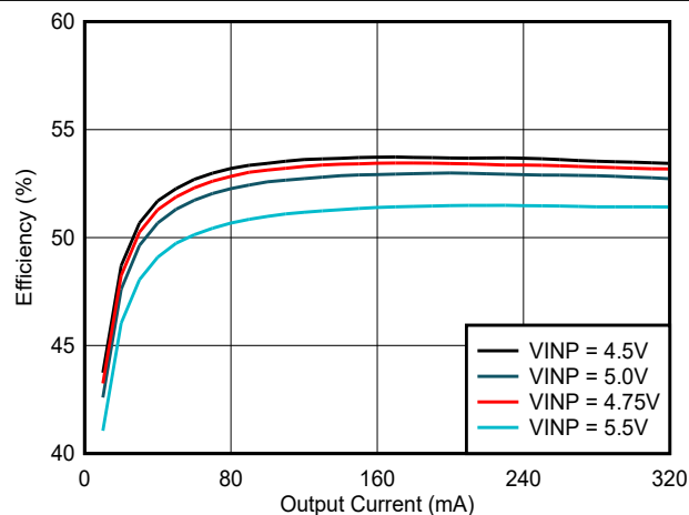
図 6-9. 効率と負荷電流 ( I_{VCC} ) との関係 : V_{CC} = 3.7V , T_A = 25^\circ C , C_{OUT2} = 22\mu F
