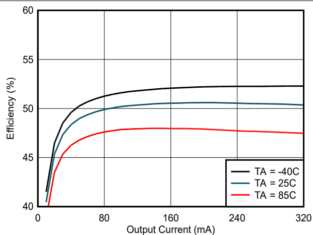
図 6-8. 効率と負荷電流 ( I_{VCC} ) との関係 : V_{CC} = 3.3V , V_{INP} = 5.0V , C_{OUT2} = 22\mu F
