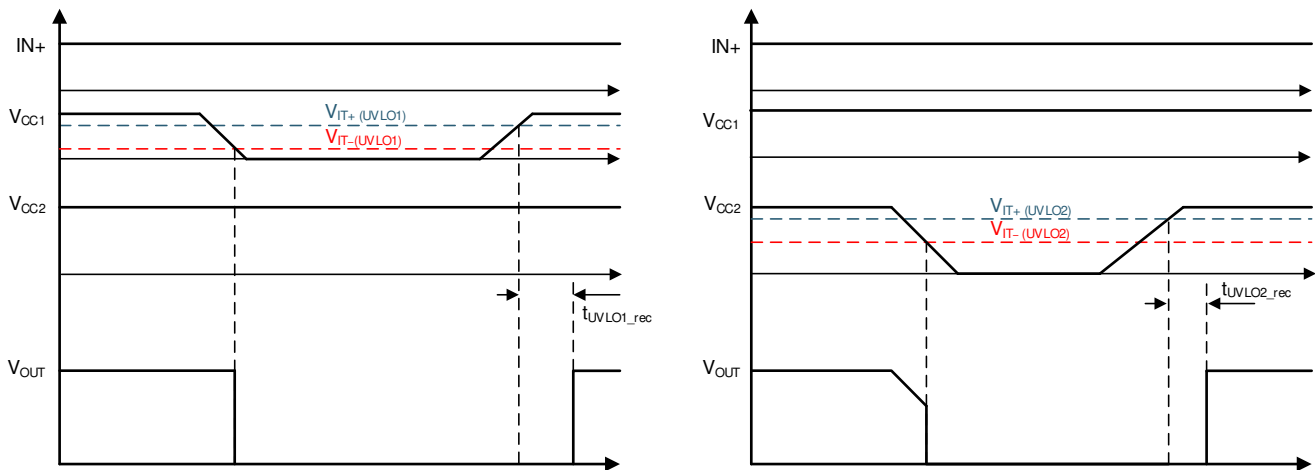
図 8-7. UVLO Functions
