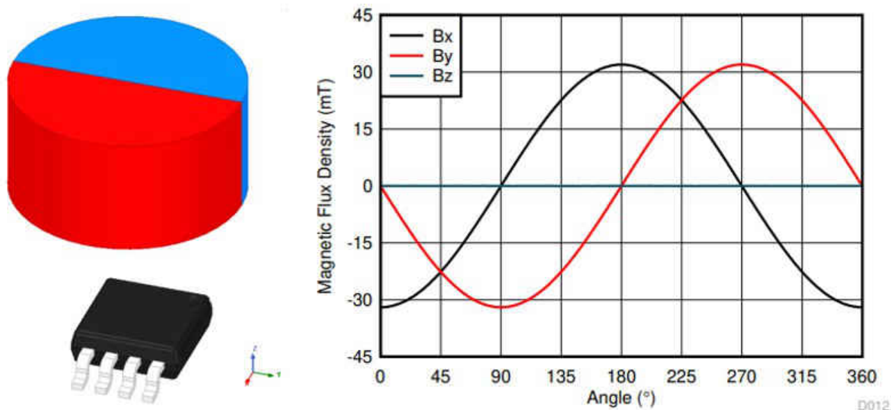
図 2-5. 3D リニア・ホール・エフェクト・センサの磁石と出力データ
