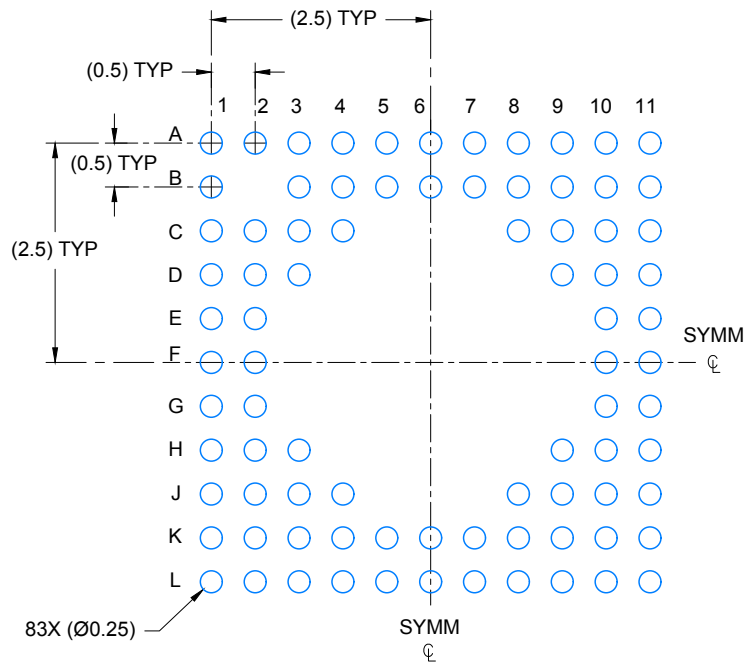
LAND PATTERN EXAMPLE SCALE: 12X
