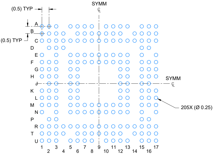
LAND PATTERN EXAMPLE SCALE: 8X
