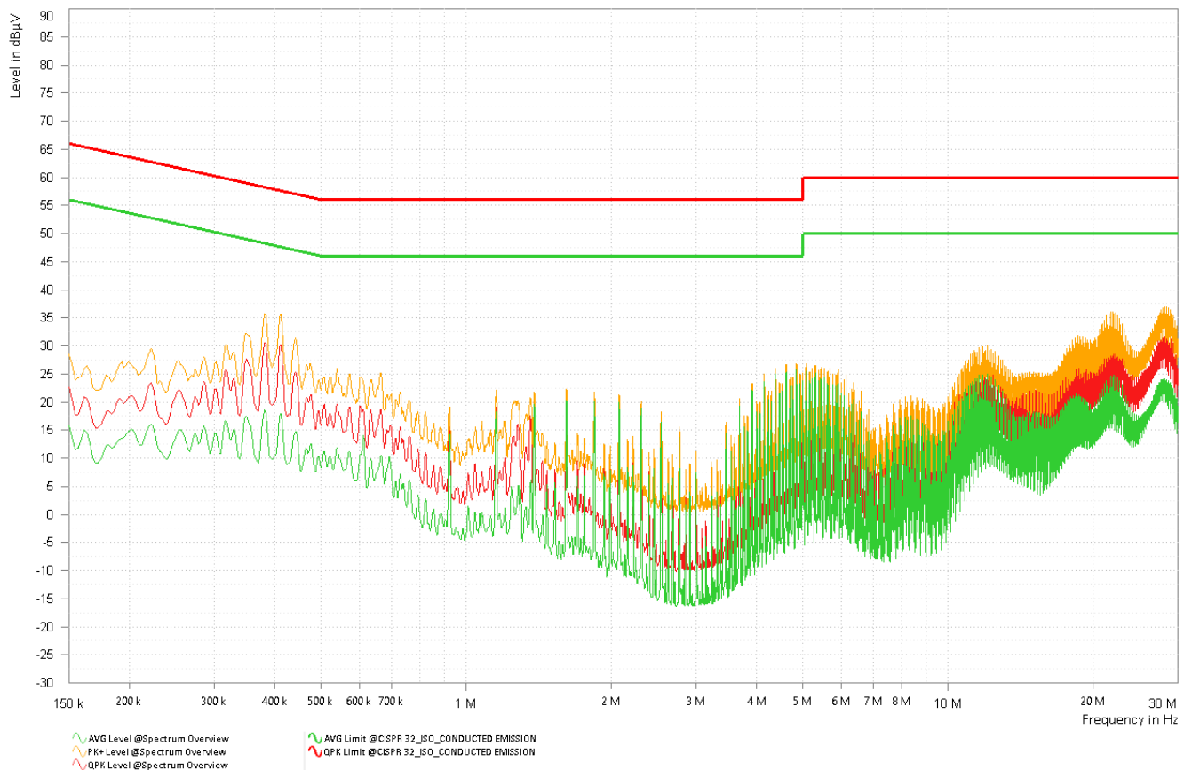
図 3-8. CISPR 32 Class B 伝導エミッション データ (VDD (ピン 1))
