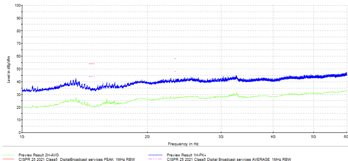
図 3-5. ISOW64xx デバイスの CISPR 25 Class 5 放射エミッション データを 1GHz から 6GHz に
