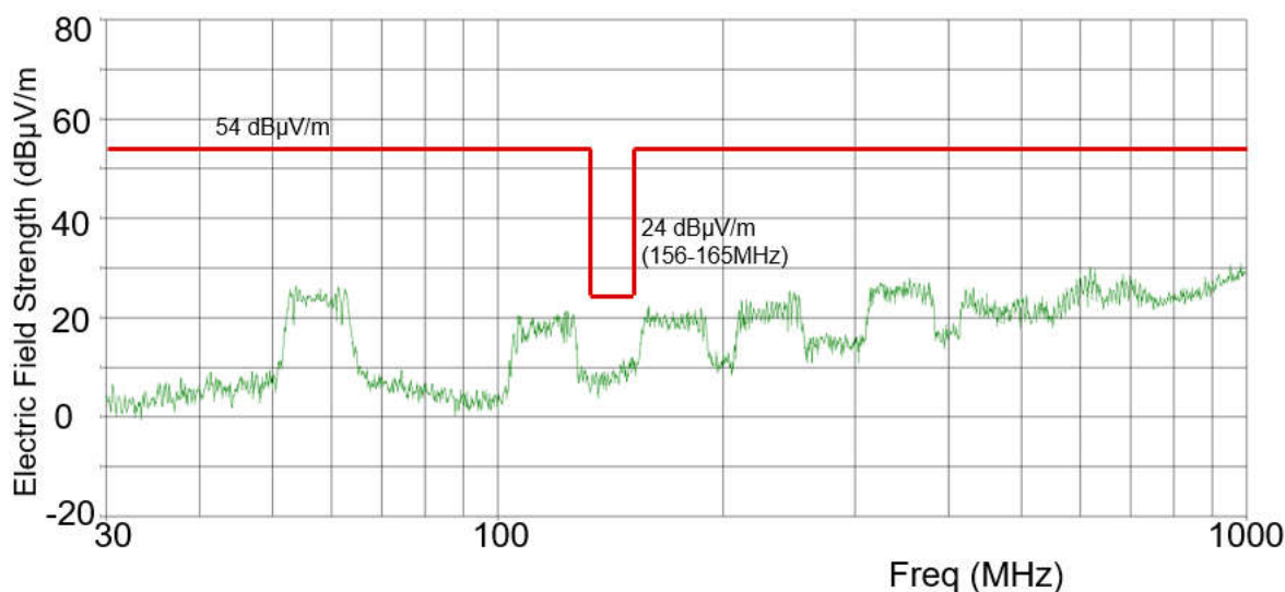
図 3-6. 30MHz ~ 1000MHz 5V5 モード (110mA 負荷) における準ピーク放射エミッション データ
