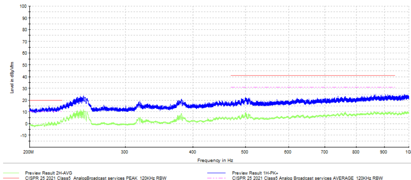
図 3-4. ISOW64xx デバイスの CISPR 25 Class 5 放射エミッション データを 200MHz から 1GHz に
