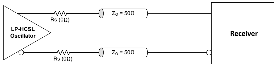
図 4-3. LP - HCSL 出力終端
