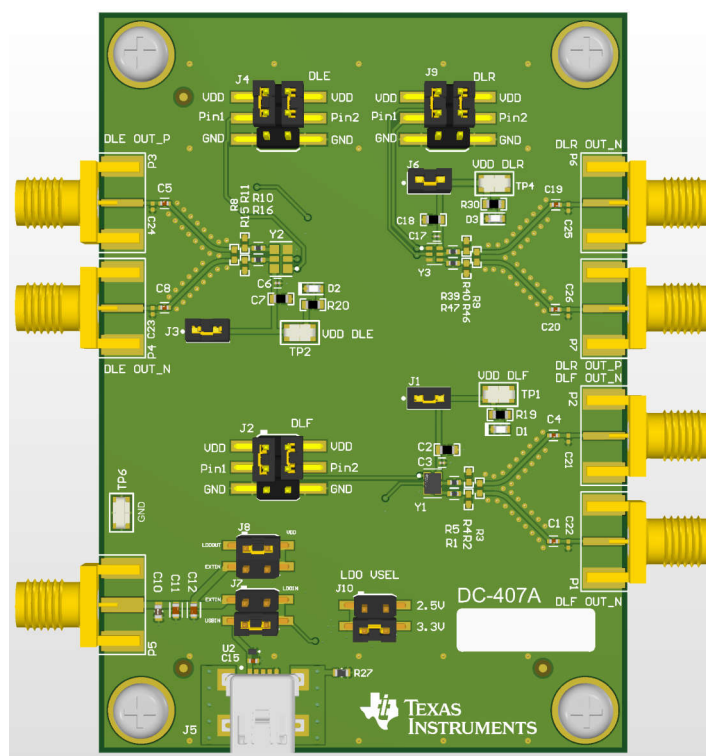
LMK6LEVM 評価ボード
