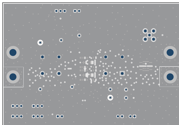
図 5-6. 内層 3
