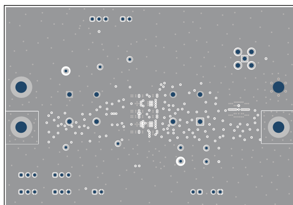
図 5-4. 内層 1
