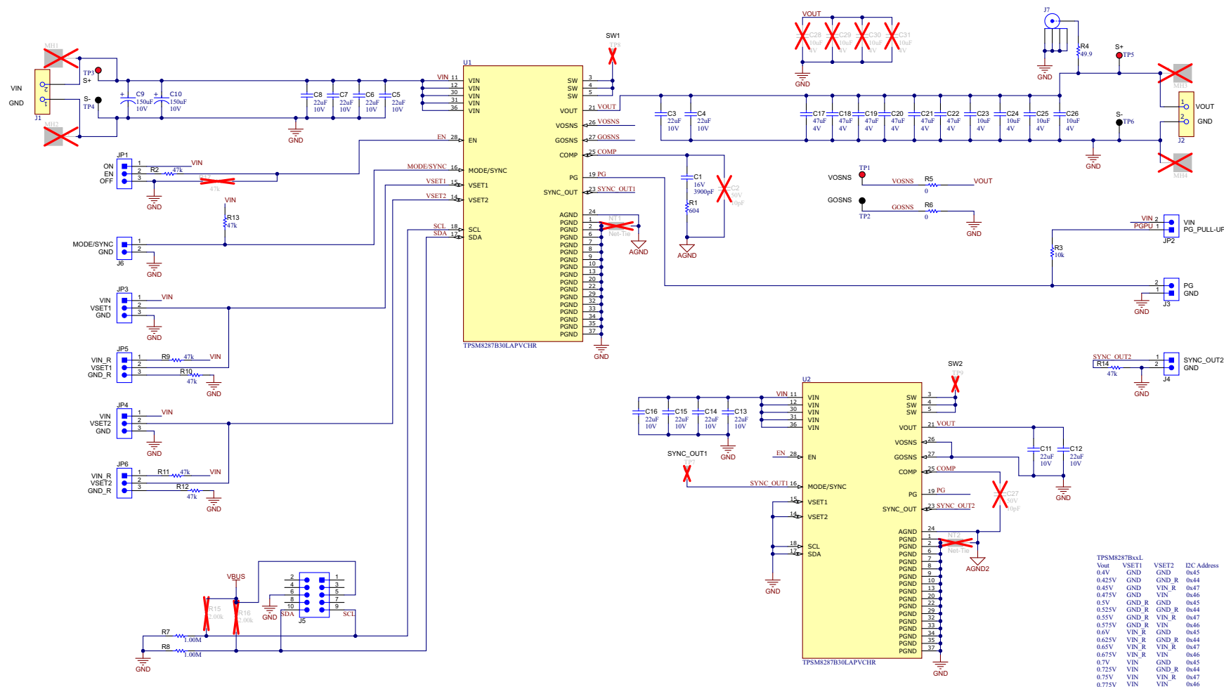
図 5-1. TPSM8287B30-2X-EVM の回路図
