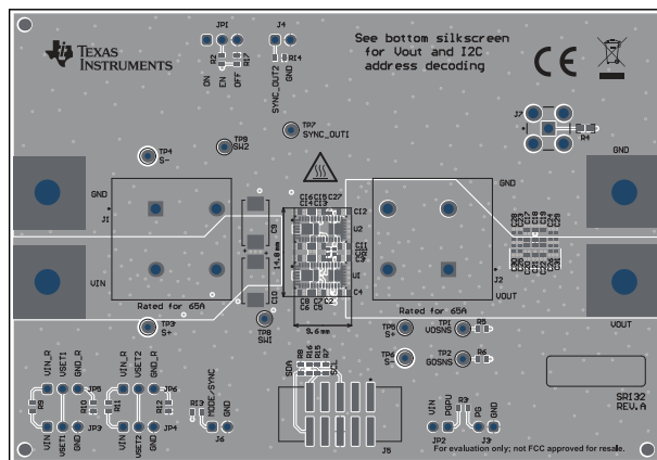
図 5-2. 上部アセンブリ
