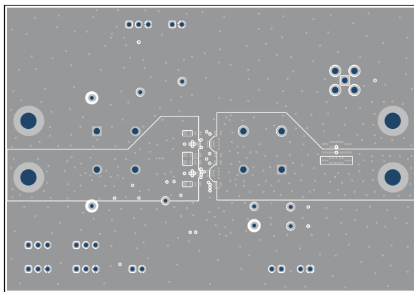
図 5-8. 内層 5
