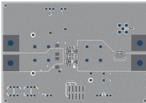
図 5-3. 上層
