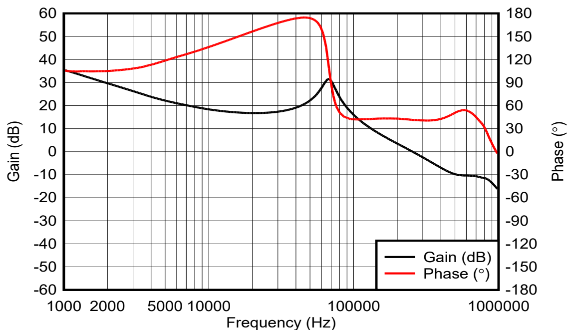
図 4-2. ループ応答の測定 (TPSM8287B30-2X-EVM, V_{IN} = 5V 、 V_{OUT} = 0.6V 、 I_{OUT} = 60A )
