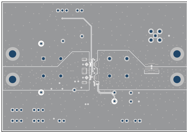
図 5-9. 内層 6
