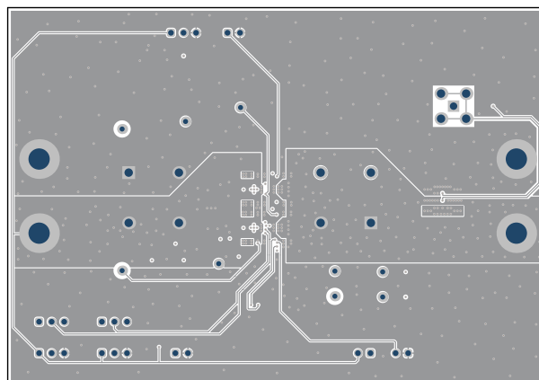
図 5-7. 内層 4
