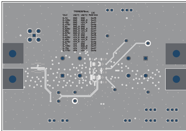
図 5-11. 下層アセンブリ (ミラーリング)
