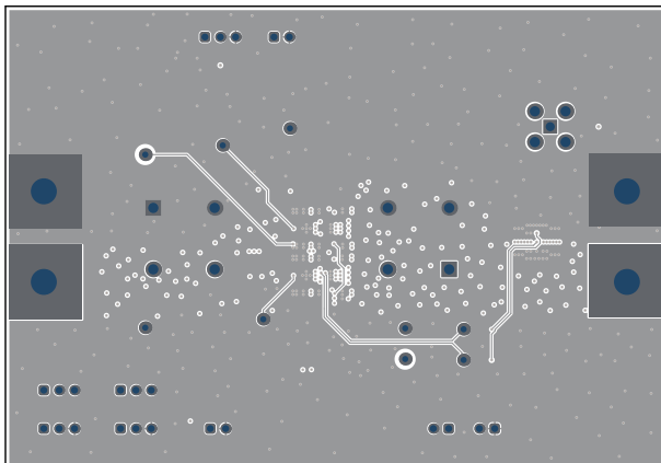
図 5-10. 下層
