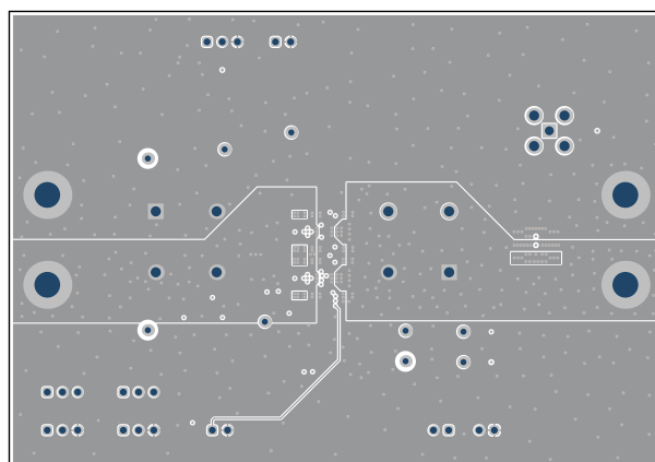
図 5-5. 内層 2
