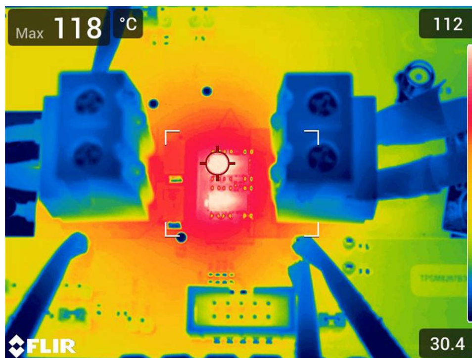
図 4-1. 放熱特性 (TPSM8287B30-2X-EVM, V_{IN} = 5V 、 V_{OUT} = 0.6V 、 I_{OUT} = 60A )
