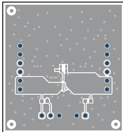
図 3-3. 上層
