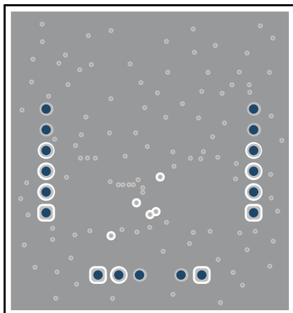
図 3-4. 信号層 1
