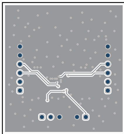
図 3-6. 下層
