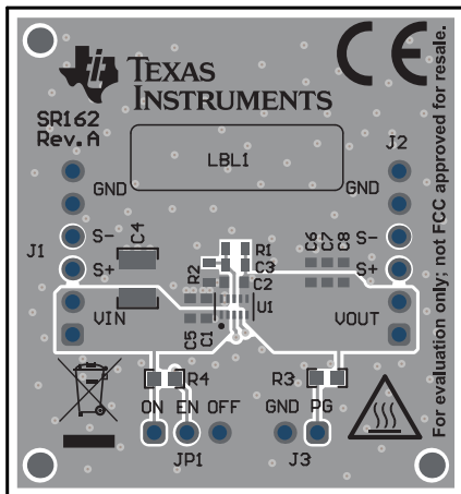
図 3-2. 上部アセンブリ
