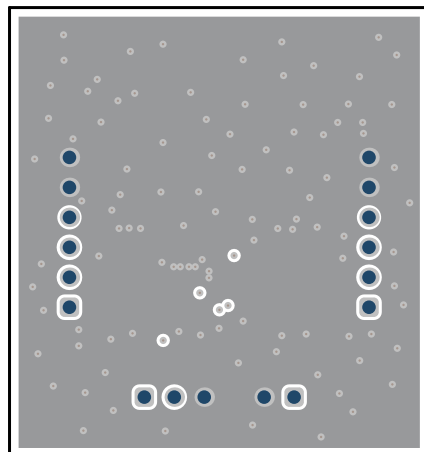
図 3-5. 信号層 2
