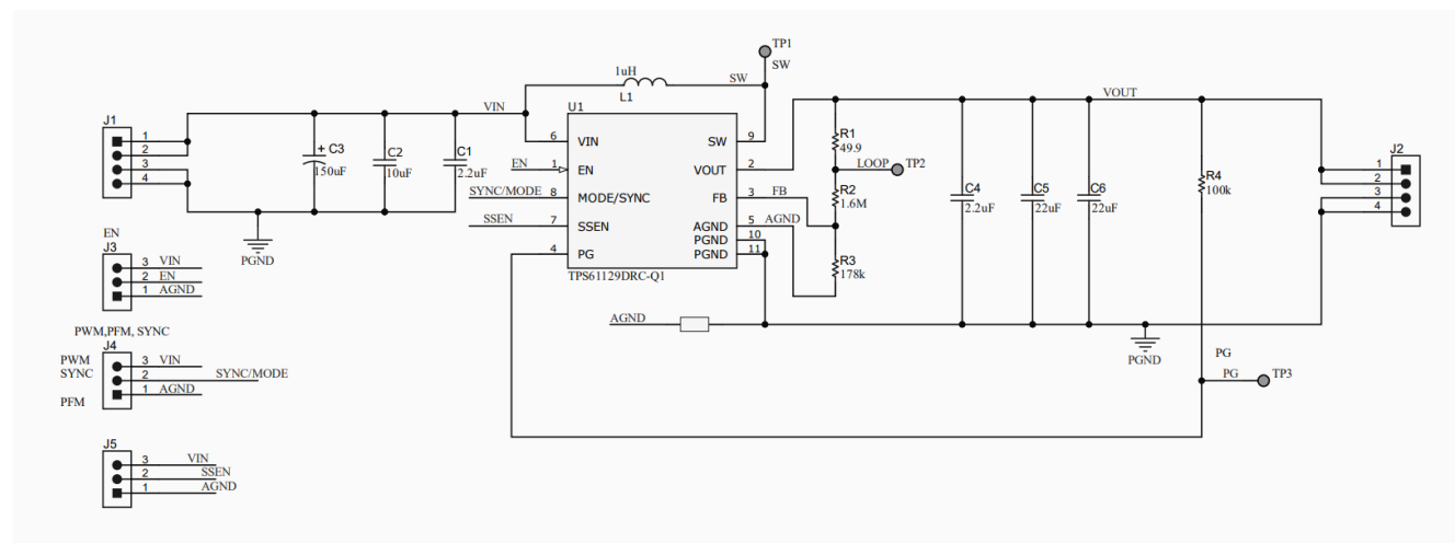
図 3-1. 回路図
