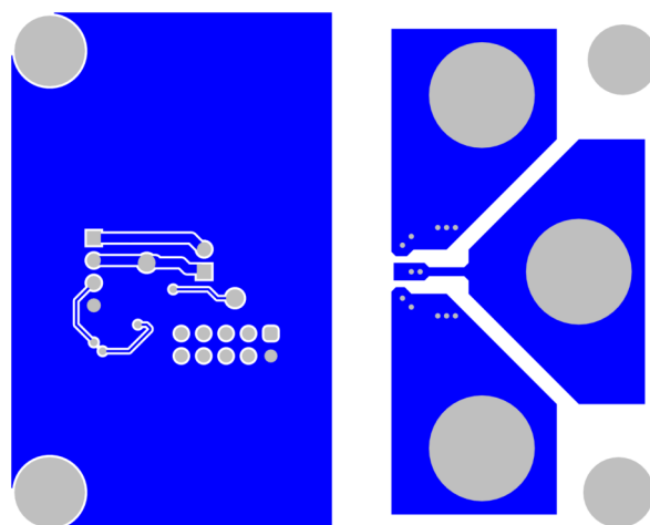
図 4-4. TPSI88XXEVM 最下層
