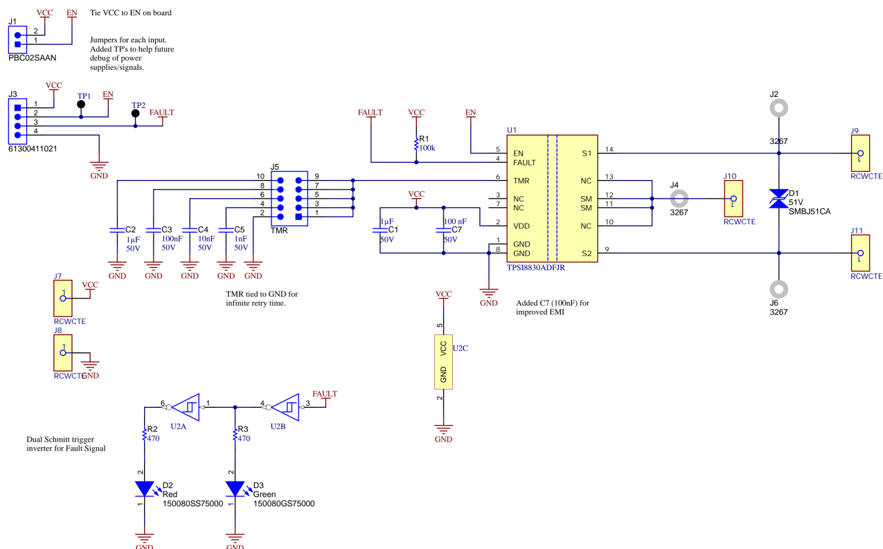
図 4-1. TPSI88XXEVM の回路図
