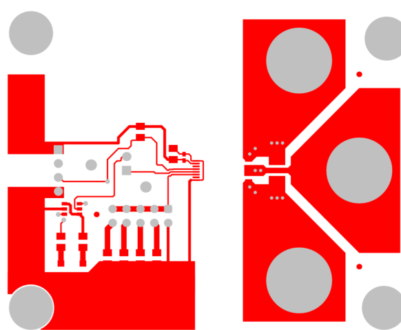
図 4-3. TPSI88XXEVM 最上層
