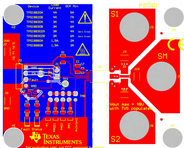
図 4-2. TPSI88XXEVM 合成図
