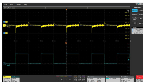
図 3-55. V_{OUT} = 12V オーバーシュート / アンダーシュート = 225mV / -463mV における負荷過渡応答
