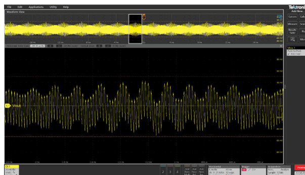
図 3-51. 全負荷時の V_{OUT} = 5V の標準リップル電圧 (104mVpp)
