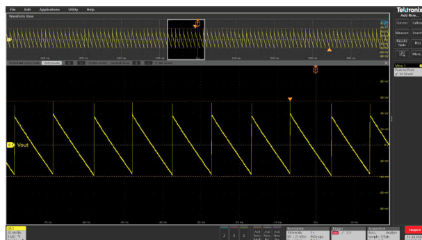
図 3-50. 無負荷時 V_{OUT} = 5V の標準リップル電圧 (95mVpp)
