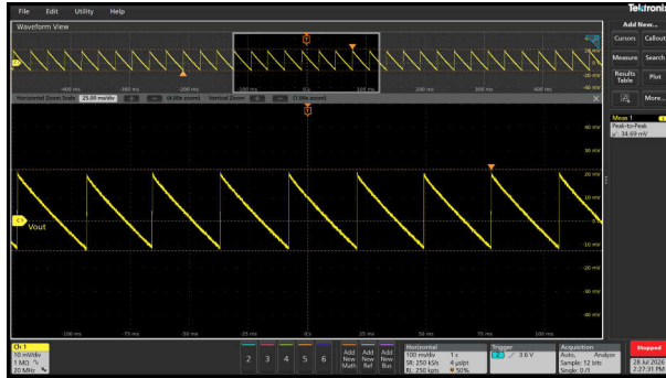
図 3-40. 無負荷時 V_{OUT} = 24V の標準リップル電圧 (35mVpp)
