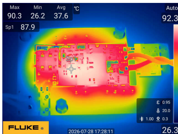
図 3-75. 230Vac ~ 24V/2.71A (底面図)
