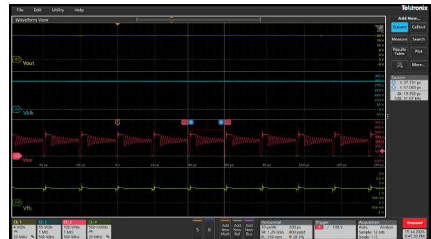
図 3-37. 230Vac/16W (52kHz 周波数 - フォールドバック / Vfb - 1.46V)
