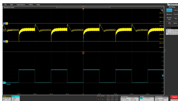
図 3-54. V_{OUT} = 15V オーバーシュート / アンダーシュート = 312mV / -523mV における負荷過渡応答
