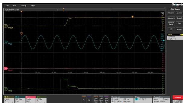
図 3-64. 24V、0A での起動応答
