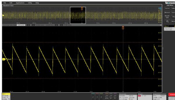
図 3-42. 無負荷時 V_{OUT} = 20V の標準リップル電圧 (55mVpp)
