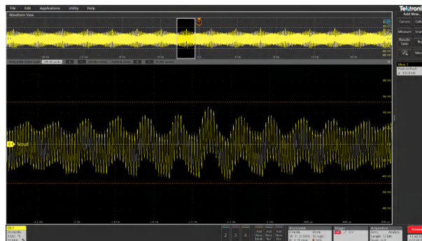
図 3-49. 全負荷時の V_{OUT} = 9V の標準リップル電圧 (102mVpp)
