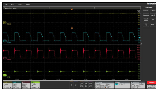
図 3-14. V_{in} = 90\text{Vac} 、 V_{out} = 20\text{V}
