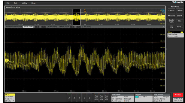
図 3-41. 全負荷時の V_{OUT} = 24V の標準リップル電圧 (112mVpp)
