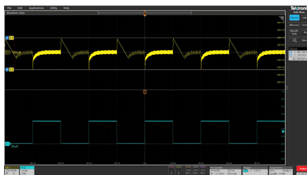
図 3-57. V_{OUT} = 5V オーバーシュート / アンダーシュート = 390mV / -458mV における負荷過渡応答
