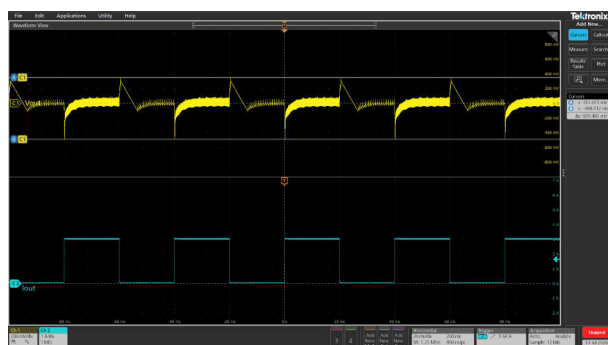
図 3-56. V_{OUT} = 9V オーバーシュート / アンダーシュート = 351mV / -488mV における負荷過渡応答
