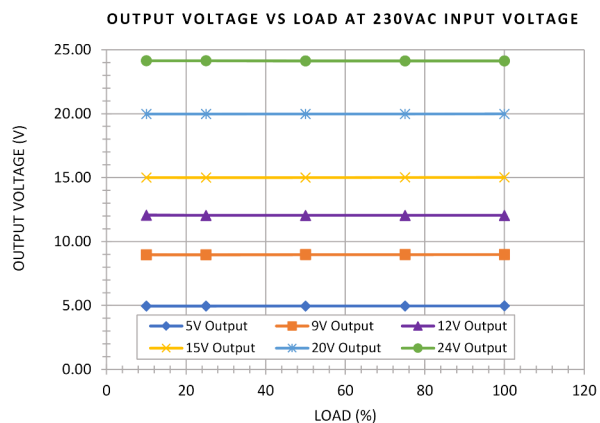
図 3-9. V_{OUT} と 230Vac 入力電圧時負荷との関係
