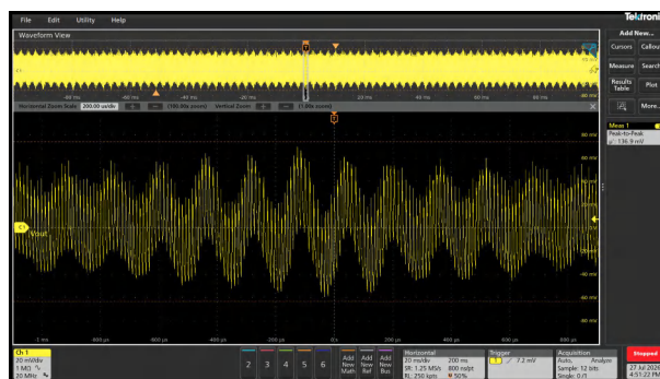
図 3-47. 全負荷時の V_{OUT} = 12V の標準リップル電圧 (137mVpp)
