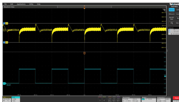
図 3-53. V_{OUT} = 20V オーバーシュート / アンダーシュート = 308mV / -566mV における負荷過渡応答
