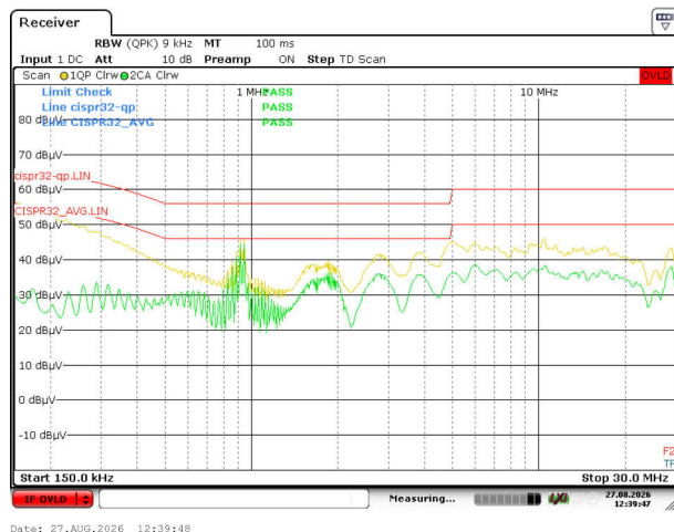
図 3-88. V_{IN} = 230V_{RMS} 、 V_{OUT} = 20V 、 I_{OUT} = 0.325A のライン
