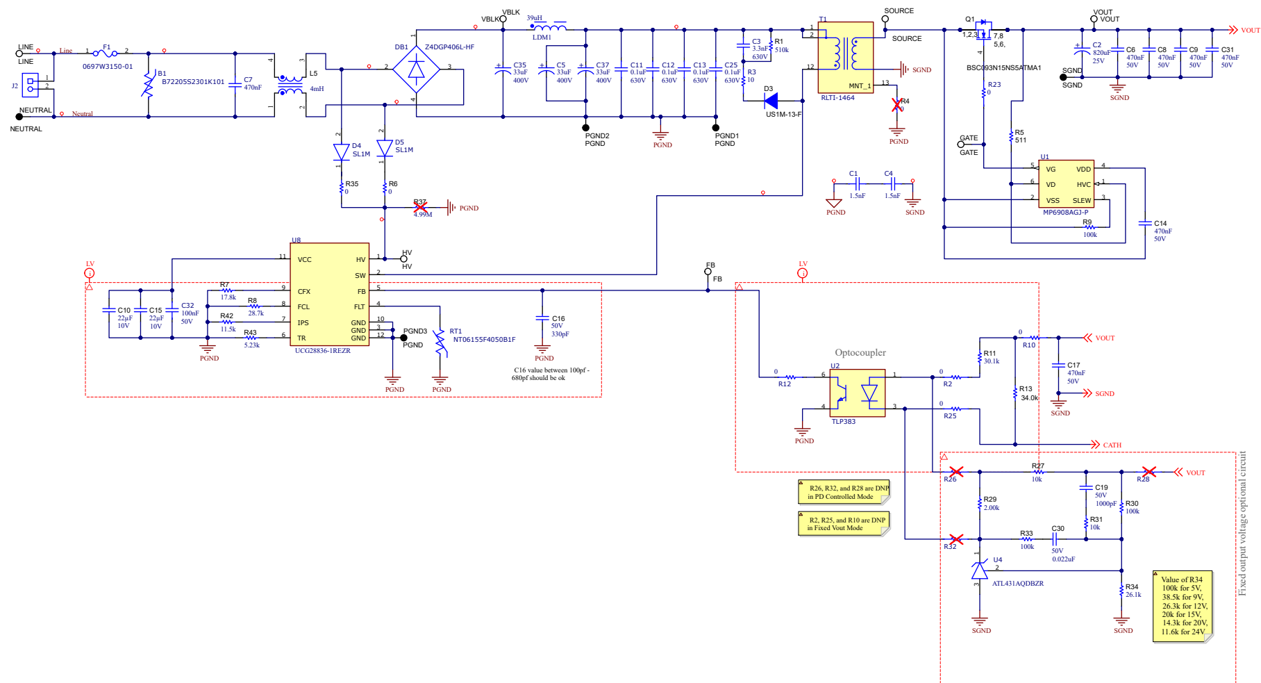
図 4-1. UCG28836EVM-150 電源回路図
