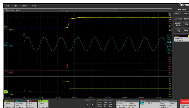
図 3-69. 5V、3A での起動応答
