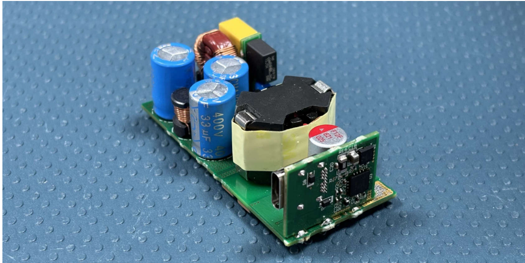
図 2-1. 高電力密度構成 (6.21cm × 2.87cm × 1.8cm)
