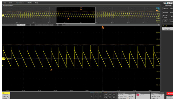
図 3-44. 無負荷時 V_{OUT} = 15V の標準リップル電圧 (75mVpp)
