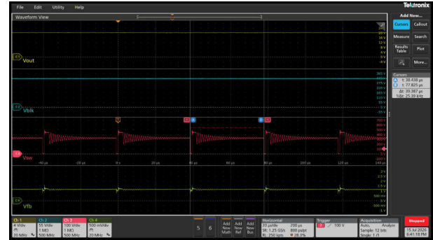
図 3-35. 230Vac/ 4.4W (25kHz 周波数 - フォールドバック / Vfb - 1.15V)
