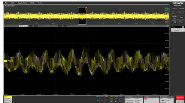
図 3-45. 全負荷時の V_{OUT} = 15V の標準リップル電圧 (103mVpp)
