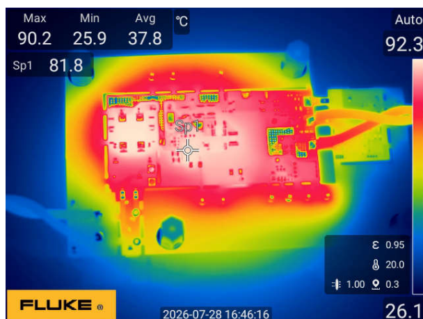
図 3-73. 115Vac ~ 24V/2.71A (底面図)
