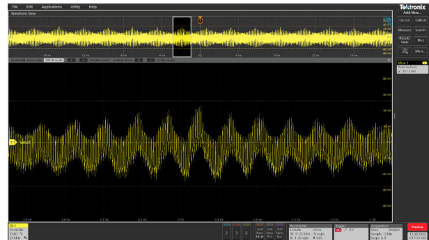
図 3-43. 全負荷時の V_{OUT} = 20V の標準リップル電圧 (108mVpp)
