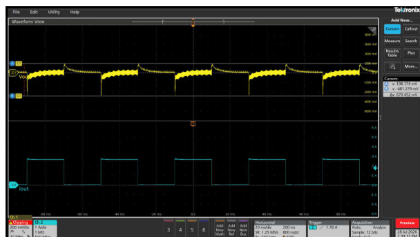
図 3-52. V_{OUT} = 24V オーバーシュート / アンダーシュート = 198mV / -481mV における負荷過渡応答
