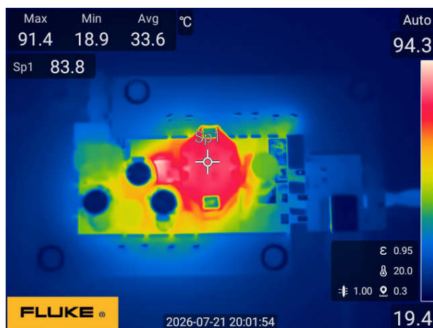
図 3-84. 264Vac ~ 20V/3.25A (上面図)
