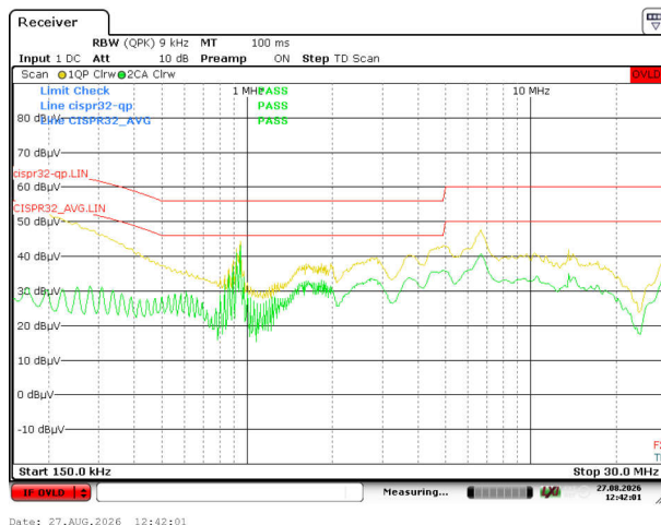
図 3-89. V_{IN} = 230V_{RMS} 、 V_{OUT} = 20V 、 I_{OUT} = 0.325A のニュートラル
