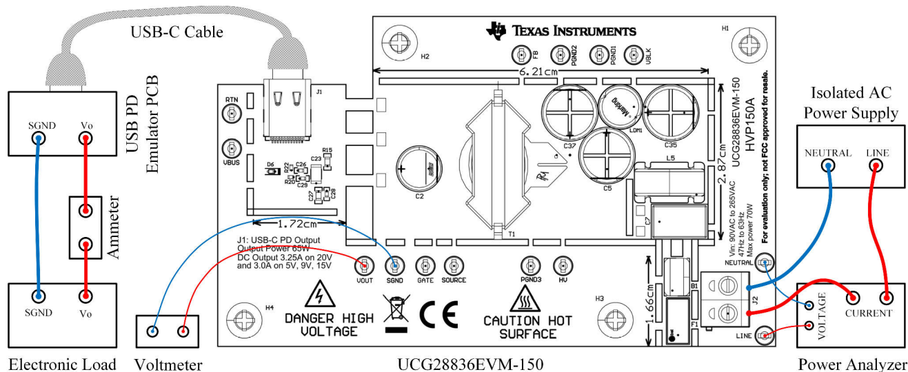
図 3-1. USB-C PD 負荷を使用した UCG28836EVM-150 のテスト設定図
