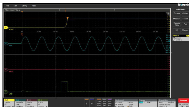
図 3-66. 12V、0A での起動応答
