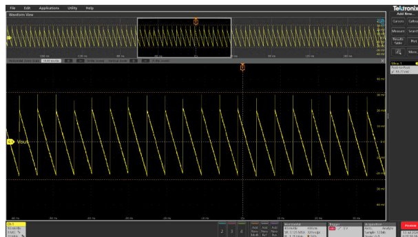
図 3-48. 無負荷時 V_{OUT} = 9V の標準リップル電圧 (56mVpp)
