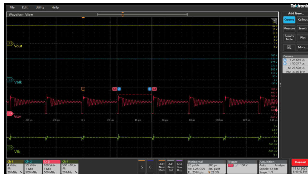
図 3-36. 230Vac/10W (39kHz 周波数 - フォールドバック / Vfb - 1.35V)
