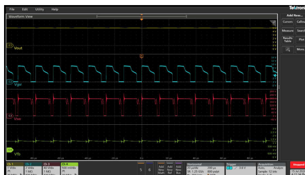
図 3-31. V_{in} = 115\text{Vac} 、 V_{out} = 5\text{V}
