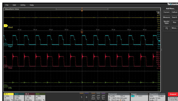
図 3-10. V_{in} = 90\text{Vac} 、 V_{out} = 24\text{V}
