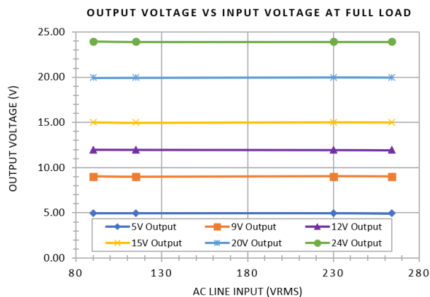
図 3-8. V_{OUT} と全負荷時入力電圧との関係
