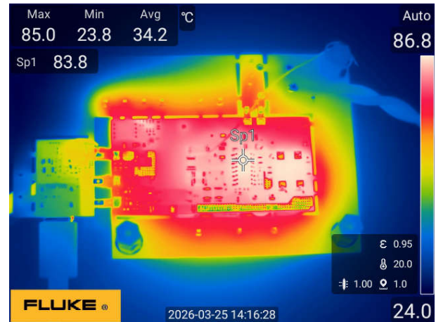
図 3-81. 115Vac ~ 20V/3.25A (底面図)
