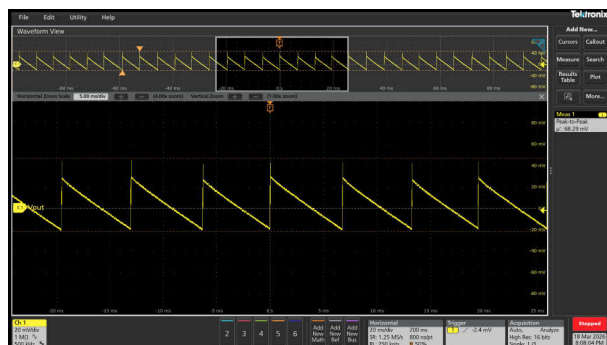
図 3-50. 無負荷時 V_{OUT} = 5V の標準リップル電圧 (68mVpp)
