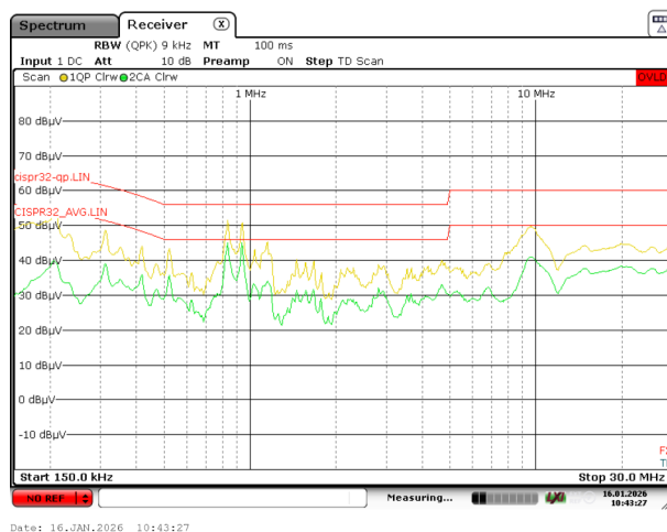
図 3-87. V_{IN} = 230V_{RMS} 、 V_{OUT} = 20V 、 I_{OUT} = 3.25A のニュートラル
