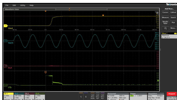
図 3-64. 24V および 0A (オーバーシュート = 230mV) での起動応答
