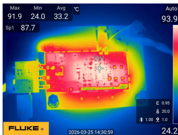
図 3-83. 230Vac ~ 20V/3.25A (底面図)
