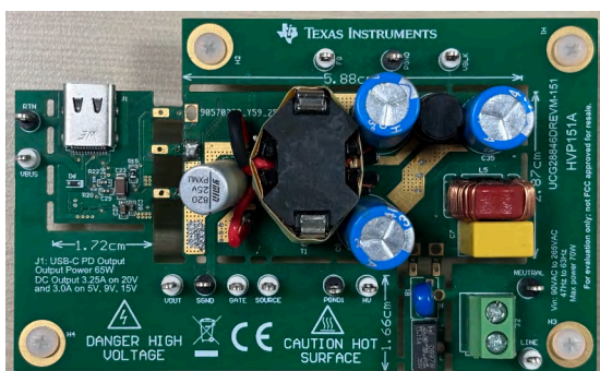
UCG28846DREVM-151 (上面図)
