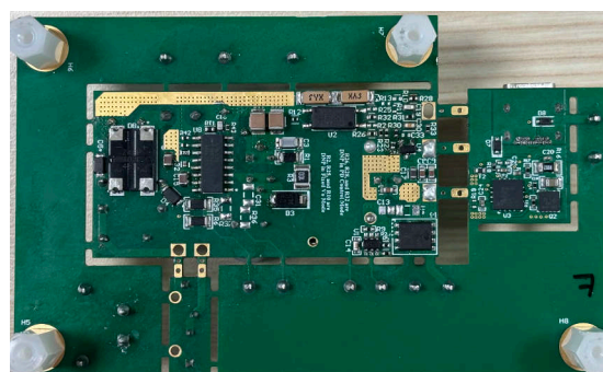
UCG28846DREVM-151 (底面図)
