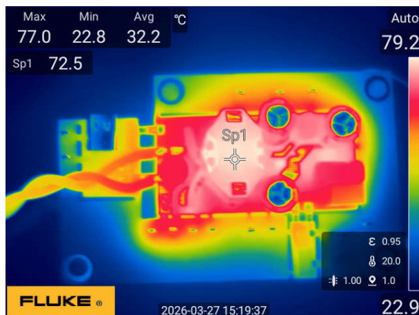
図 3-72. 115Vac ~ 24V/2.71A (上面図)
