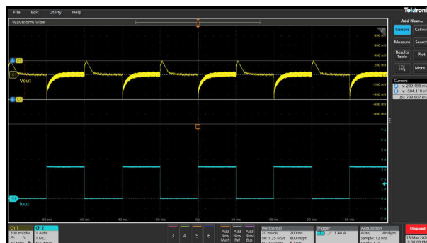
図 3-53. V_{OUT} = 20V オーバーシュート / アンダーシュート = 289mV / -504mV における負荷過渡応答
