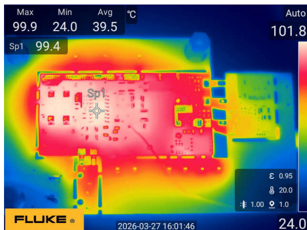
図 3-71. 90Vac ~ 24V/2.71A (底面図)
