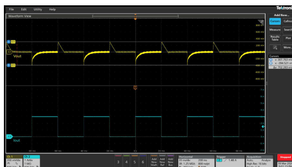
図 3-57. V_{OUT} = 5V オーバーシュート / アンダーシュート = 307mV / -395mV における負荷過渡応答
