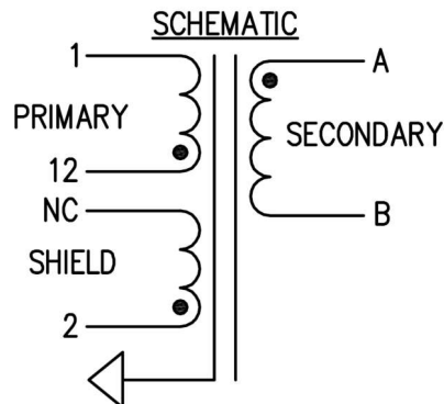
図 4-6. RLTI-1464 の回路図
