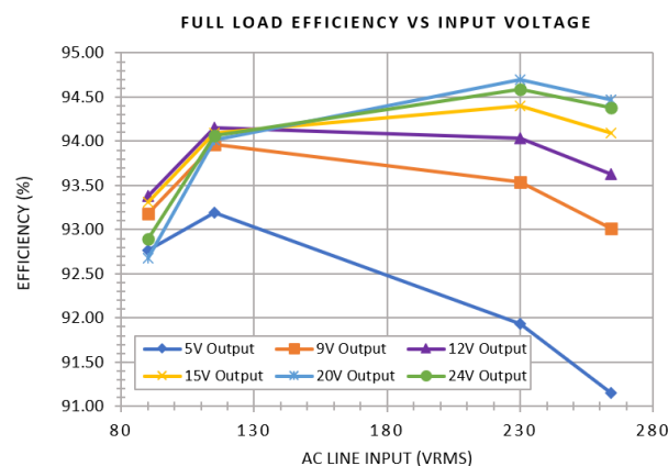
図 3-6. 全負荷効率と入力電圧との関係
