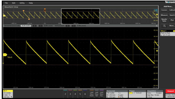
図 3-40. 無負荷時 V_{OUT} = 24V の標準リップル電圧 (42mVpp)
