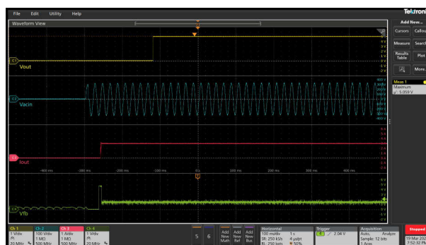
図 3-69. 5V および 3A (オーバーシュート = 59mV) での起動応答
