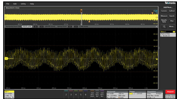
図 3-43. 全負荷時の V_{OUT} = 20V の標準リップル電圧 (86mVpp)
