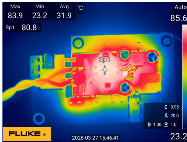
図 3-76. 264Vac ~ 24V/2.71A (上面図)
