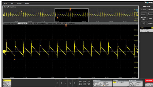
図 3-42. 無負荷時 V_{OUT} = 20V の標準リップル電圧 (74mVpp)
