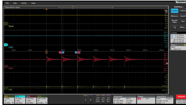
図 3-34. 230Vac/0.4W (パースト周波数 25kHz/ Vfb - 0.27V)
