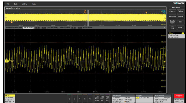
図 3-45. 全負荷時の V_{OUT} = 15V の標準リップル電圧 (98mVpp)
