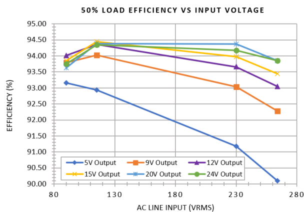
図 3-7. 50% 負荷効率と入力電圧との関係
