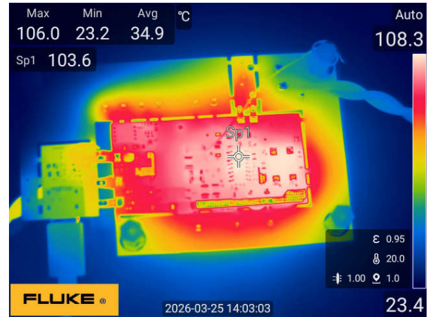
図 3-79. 90Vac ~ 20V/3.25A (底面図)
