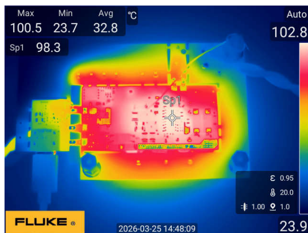
図 3-85. 264Vac ~ 20V/3.25A (底面図)
