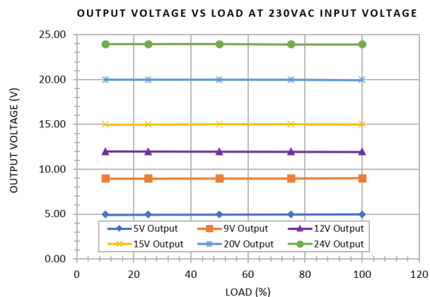
図 3-9. V_{OUT} と 230Vac 負荷時入力電圧との関係
