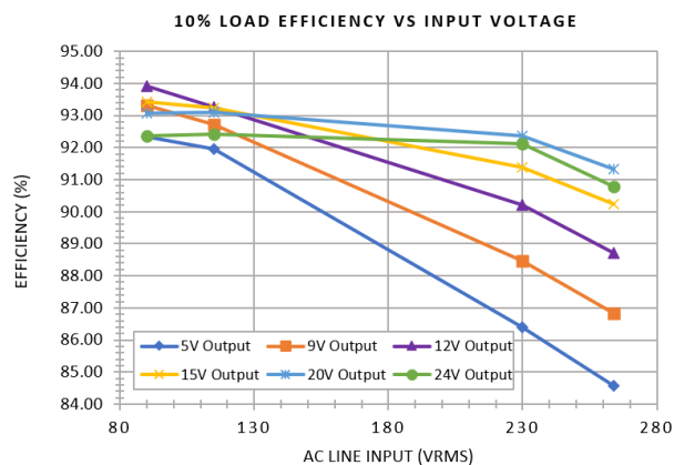
図 3-5. 10% 負荷効率と入力電圧との関係
