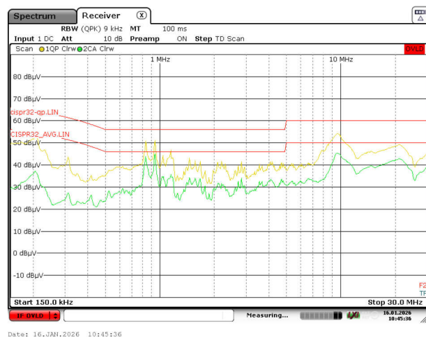
図 3-86. V_{IN} = 230V_{RMS} 、 V_{OUT} = 20V 、 I_{OUT} = 3.25A のライン
