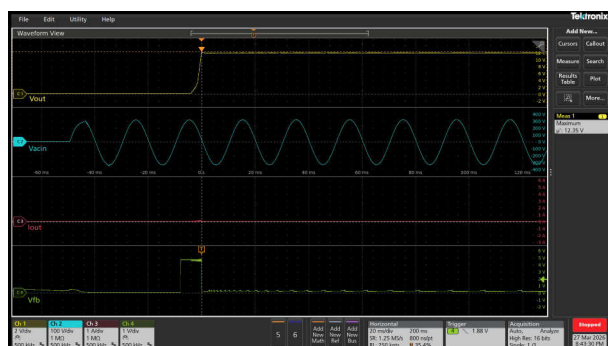
図 3-66. 12V および 0A (オーバーシュート = 350mV) での起動応答
