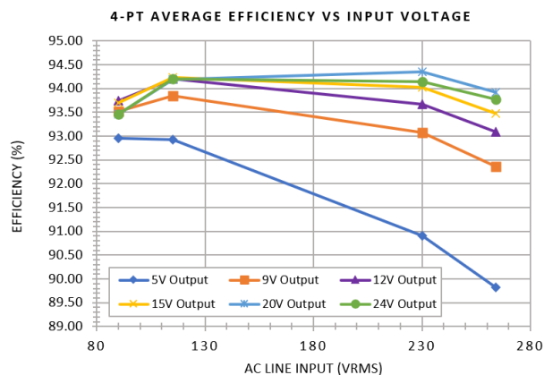
図 3-4. 4 ポイント平均効率と入力電圧との関係
