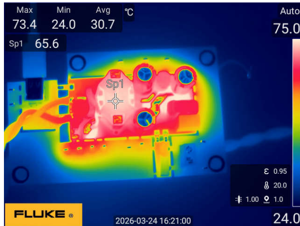
図 3-80. 115Vac ~ 20V/3.25A (上面図)
