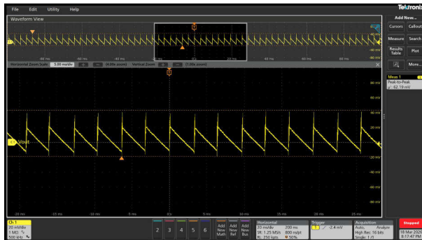
図 3-44. 無負荷時 V_{OUT} = 15V の標準リップル電圧 (62mVpp)
