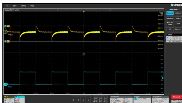
図 3-56. V_{OUT} = 9V オーバーシュート / アンダーシュート = 299mV / -449mV における負荷過渡応答
