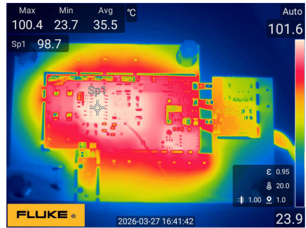
図 3-77. 264Vac ~ 24V/2.71A (底面図)
