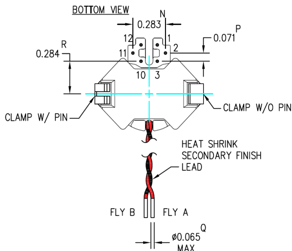
図 4-5. RLTI-1464 ピン構成
