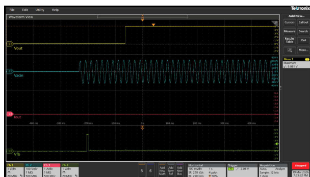
図 3-68. 5V および 0A (オーバーシュート = 61mV) での起動応答
