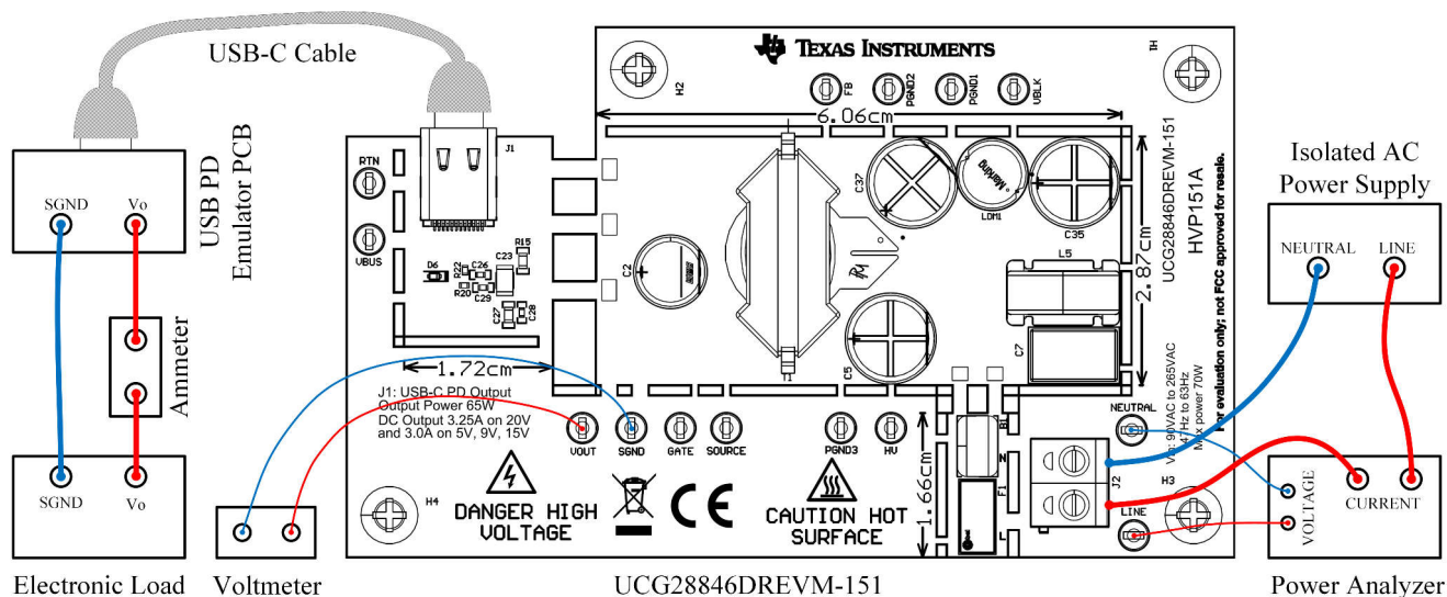
図 3-1. USB-C PD 負荷を使用した UCG28846DREVM-151 のテスト設定図
