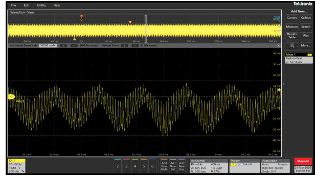
図 3-41. 全負荷時の V_{OUT} = 24V の標準リップル電圧 (50mVpp)
