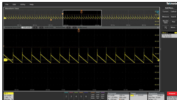
図 3-48. 無負荷時 V_{OUT} = 9V の標準リップル電圧 (52mVpp)
