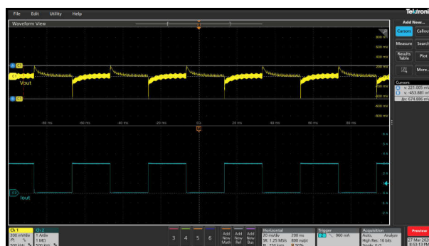
図 3-55. V_{OUT} = 12V オーバーシュート / アンダーシュート = 221mV / -454mV における負荷過渡応答
