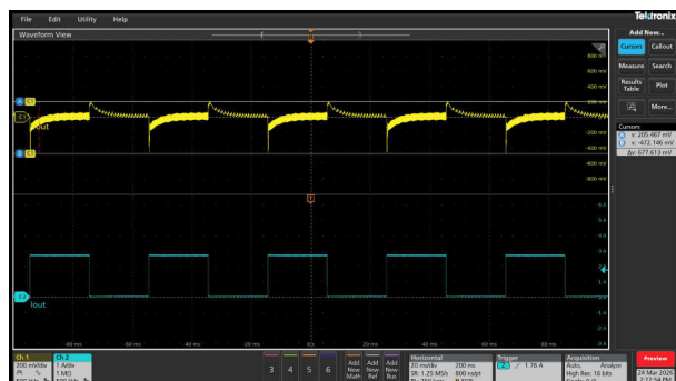
図 3-52. V_{OUT} = 24V オーバーシュート / アンダーシュート = 205mV / -472mV における負荷過渡応答
