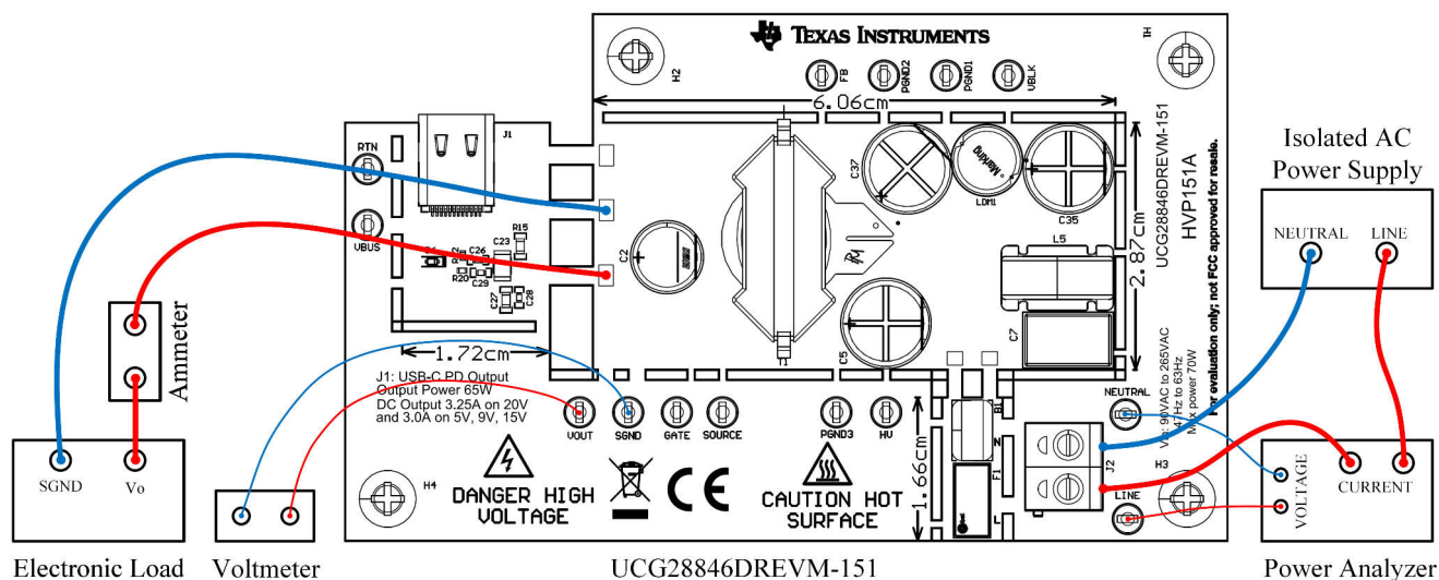
図 3-2. USB-C 以外の PD 負荷を使用した UCG28846DREVM-151 のテスト設定図
