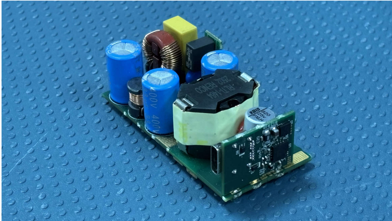
図 2-1. 高電力密度構成 (6.06cm × 2.87cm × 1.8cm)
