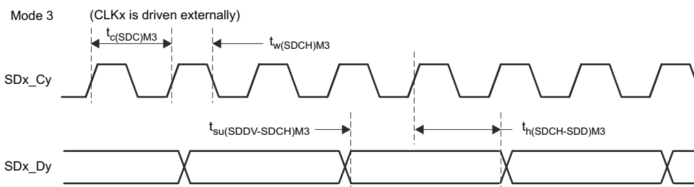
図 6-77. SDFM タイミング図 – モード 3
