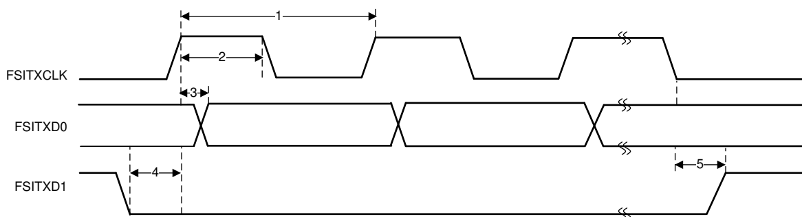
図 6-99. FSITX SPI 信号モードのタイミング
