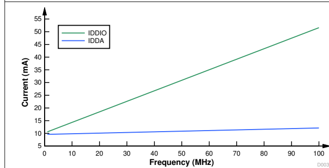
図 6-4. 電流と周波数との関係—DC/DC
