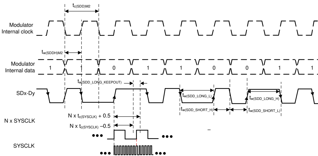
図 6-76. SDFM タイミング図 – モード 2
