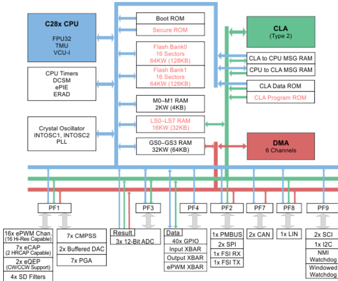
図 7-1. 機能ブロック図
