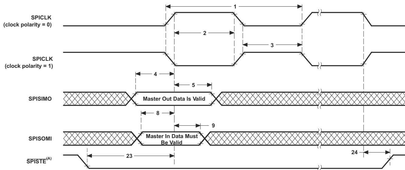
図 6-89. 高速 SPI マスタ モードの外部タイミング (クロック位相 = 1)
