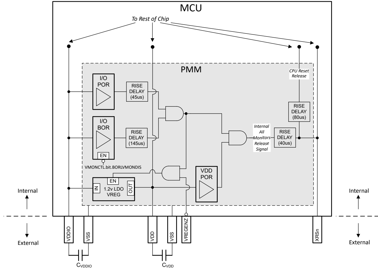
図 6-6. PMM のブロック図
