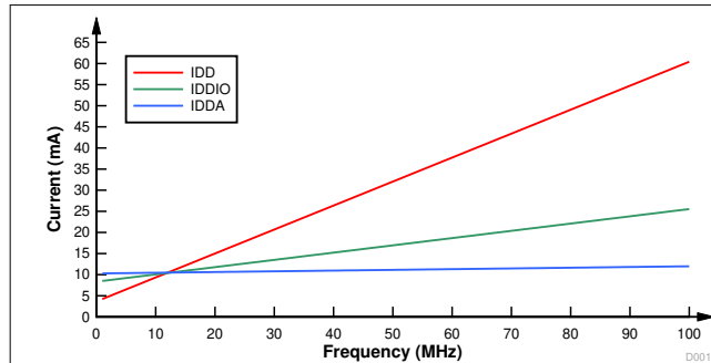
図 6-2. 電流と周波数との関係—外部電源
