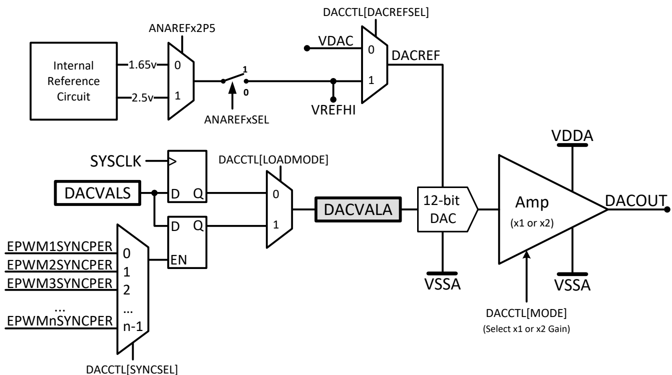
図 6-47. DAC モジュールのブロック図
