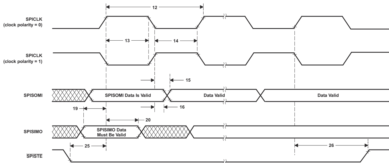
図 6-91. 高速 SPI スレーブ・モードの外部タイミング (クロック位相 = 1)
