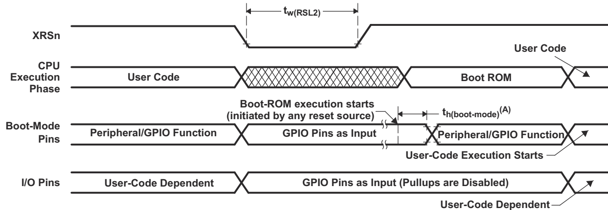
図 6-13. パワーオン・リセット
