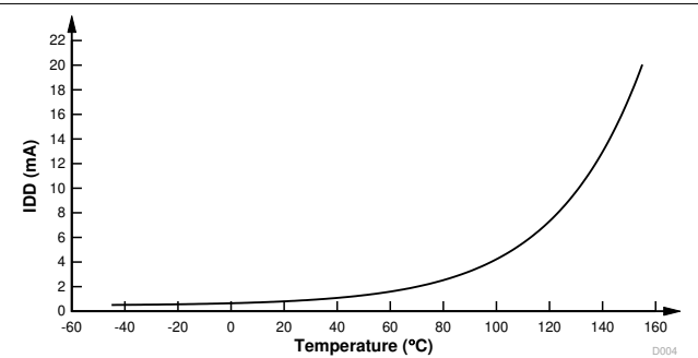
図 6-5. ホールド時の電流と温度 (°C) との関係
