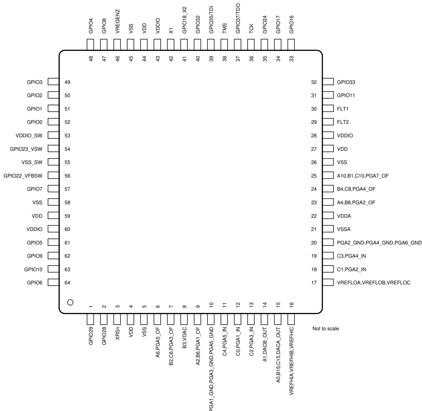
図 5-3. F280048/C、F280040/C 64 ピン PM 薄型クワッド・フラットバック - Q 温度 (上面図)
