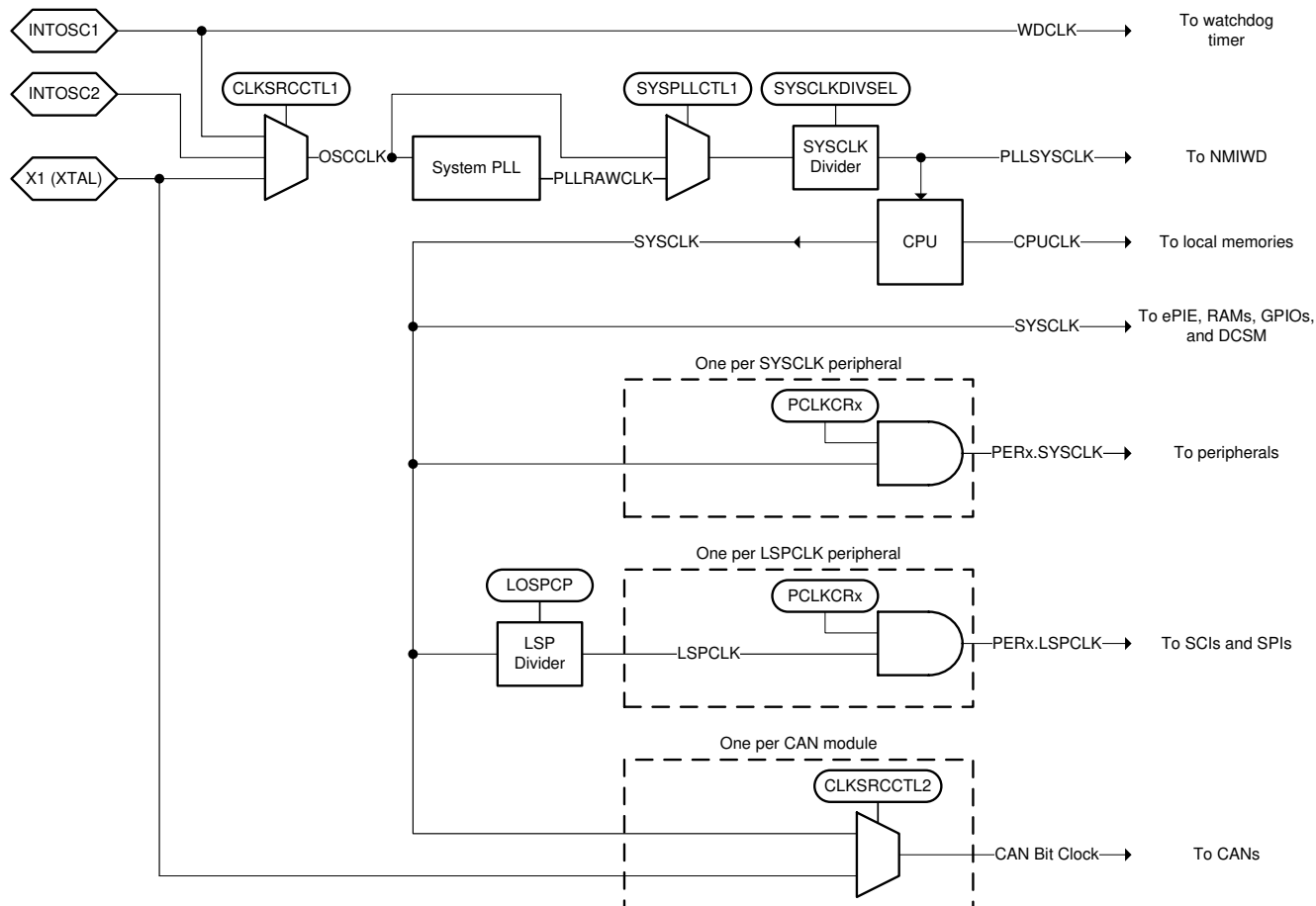
図 6-15. クロック供給システム
