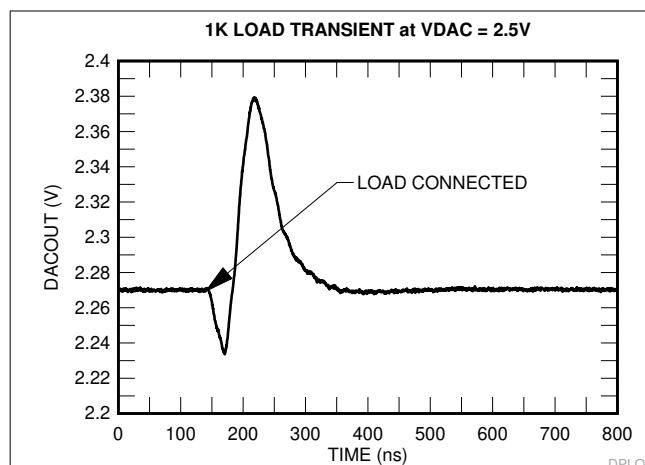
図 6-55. 1k \Omega の負荷過渡応答
