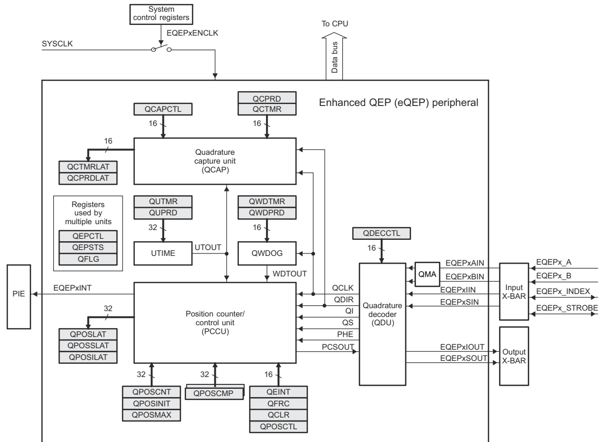
図 6-72. eQEP のブロック図
