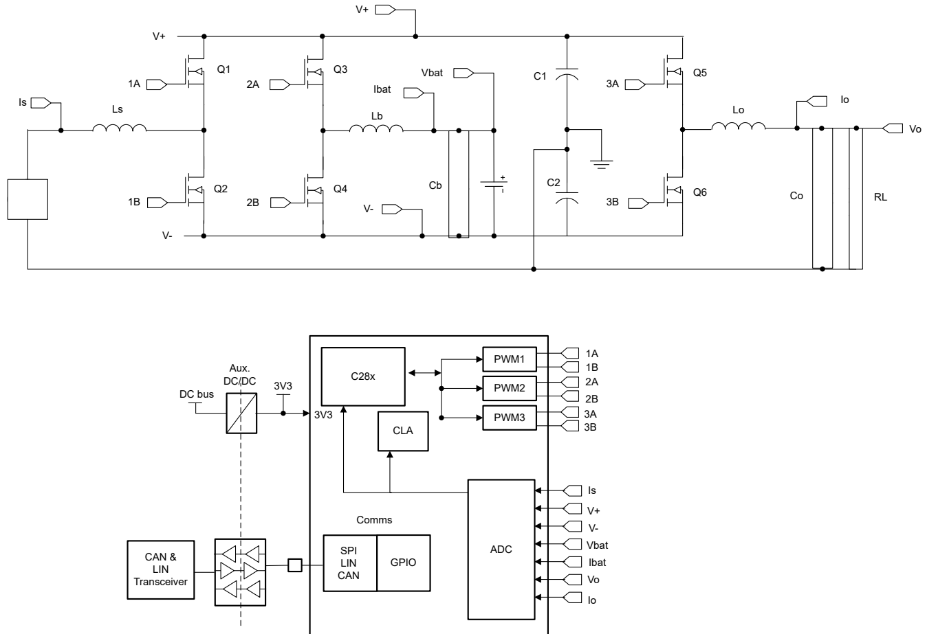
図 8-4. 単相オンライン UPS
