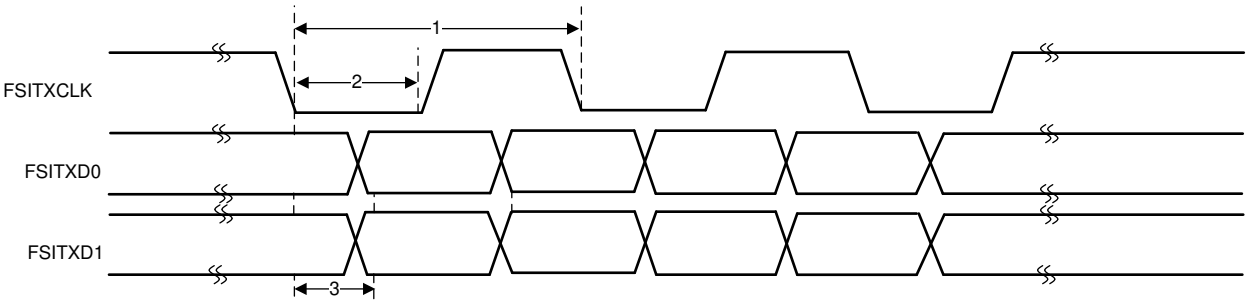
図 6-95. FSITX タイミング
