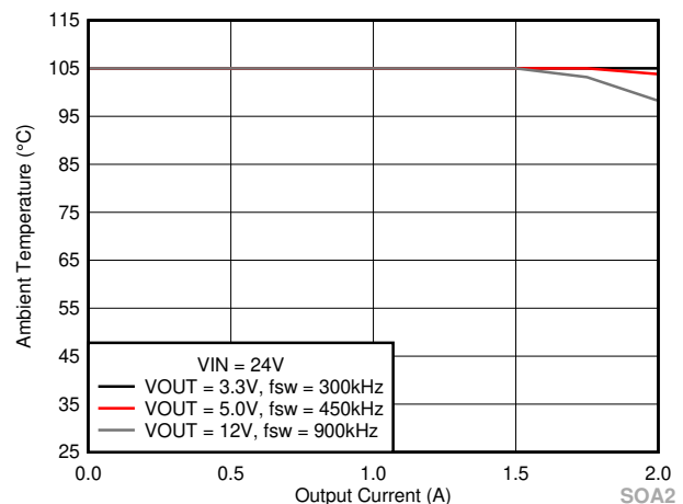
安全動作領域
