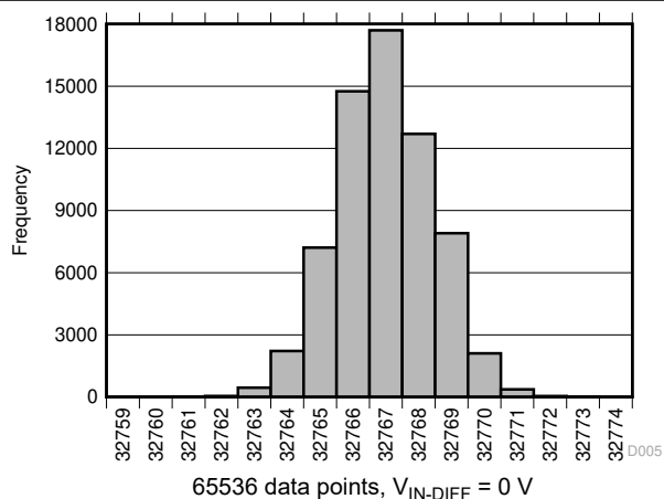
FIG 6-11. DC Histogram
