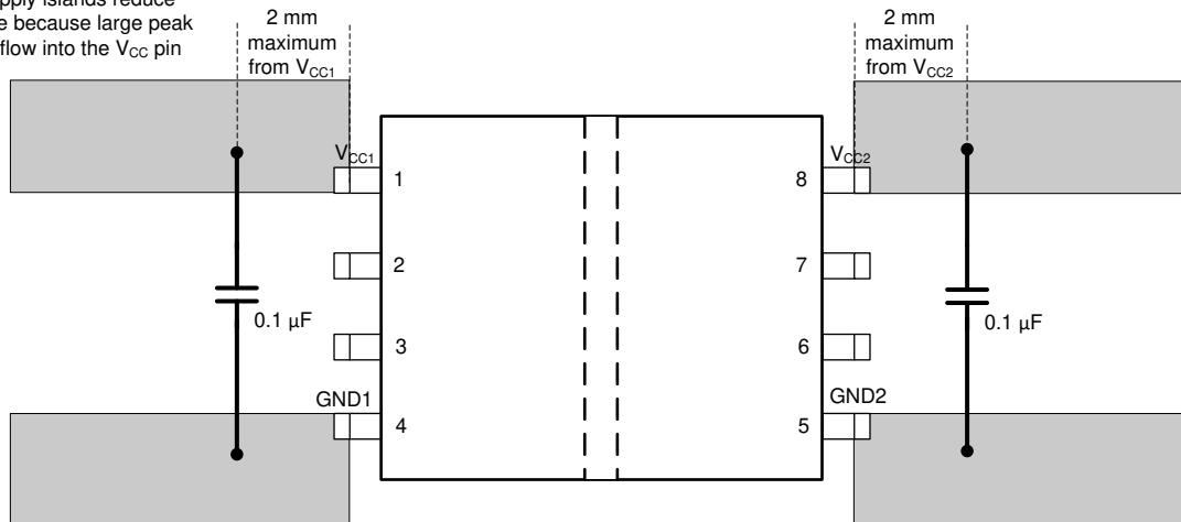
✎ 12-1. Layout Example
