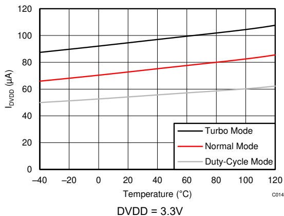
図 6-35. I_{DVDD} vs 温度
