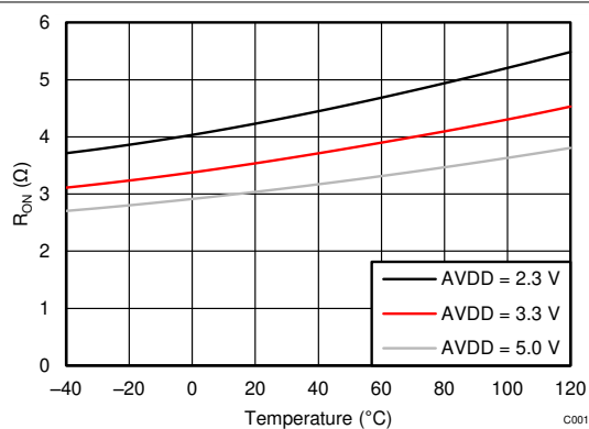
図 6-37. ローサイド パワー スイッチ R_{\text{ON}} と温度との関係
