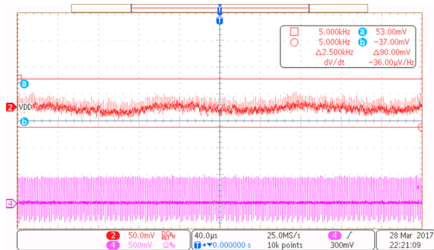
図 19. Auxiliary Rail — 10-A to 20-A Transient, 600-kHz Load Frequency
