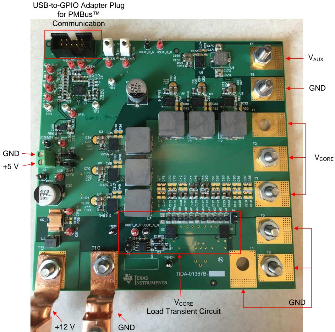
図 1. TIDA-01367 Test Setup
