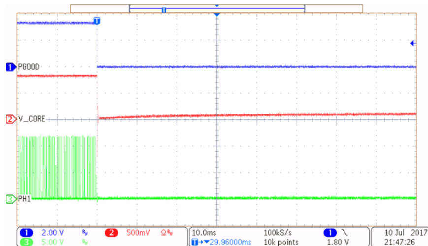
図 29. Overtemperature Shutdown
