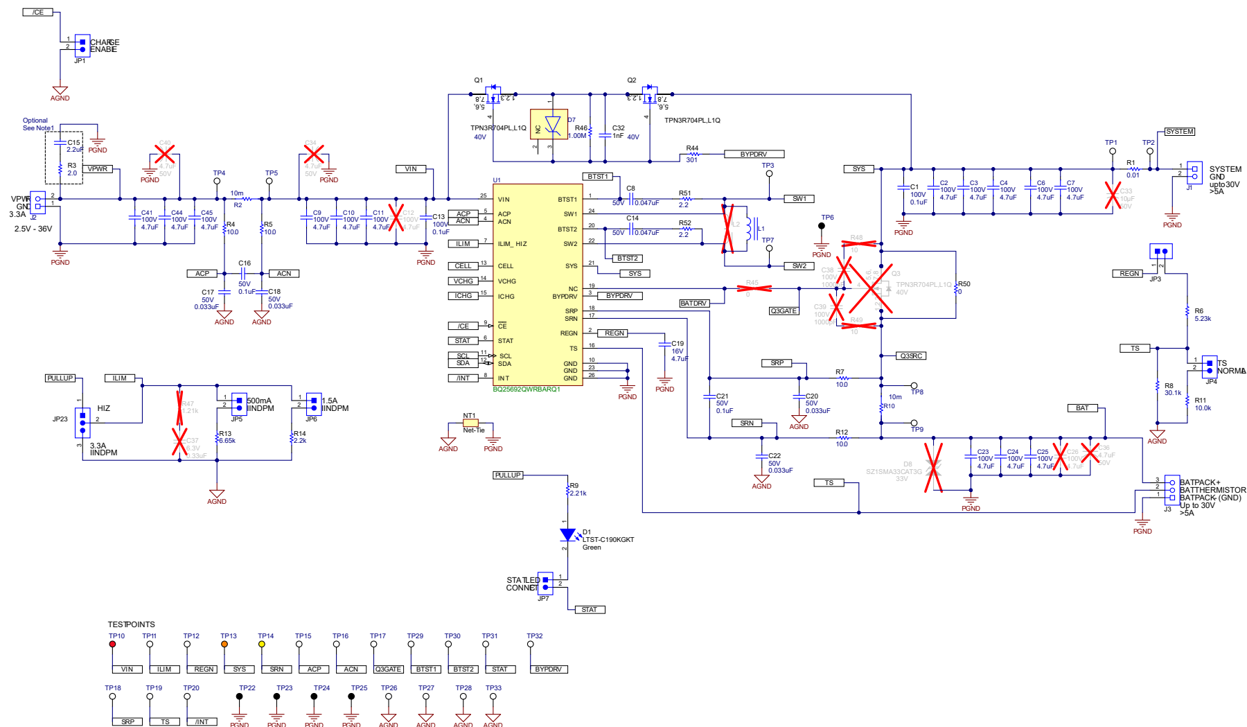
図 4-1. BQ25692-Q1EVM BMS083B 回路図ページ 1
