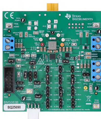
BQ2569X/9X-Q1EVM ハードウェア ボード
