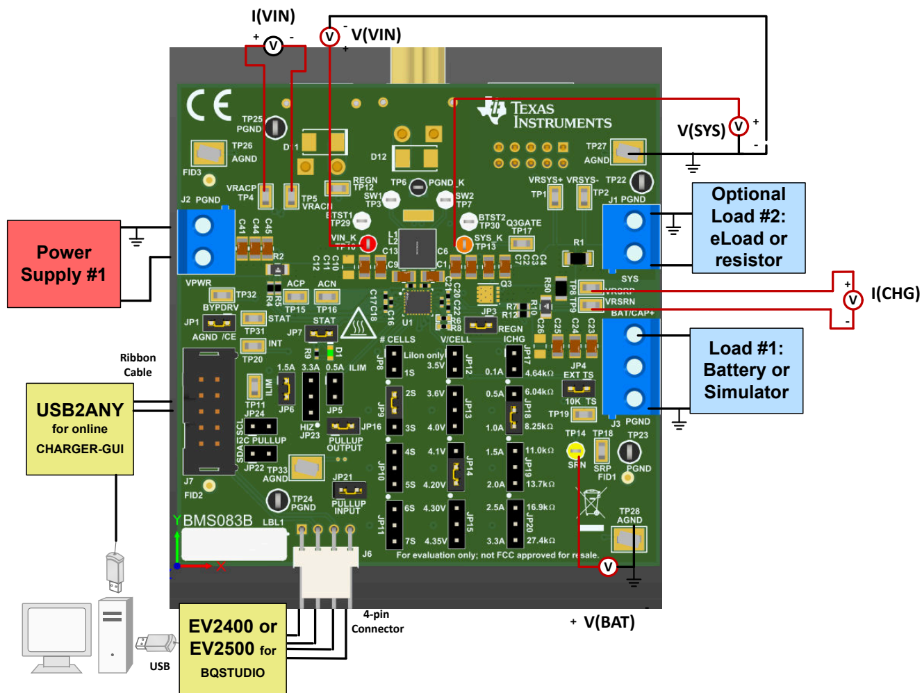
図 2-1. BQ25692-Q1EVM のテスト設定
