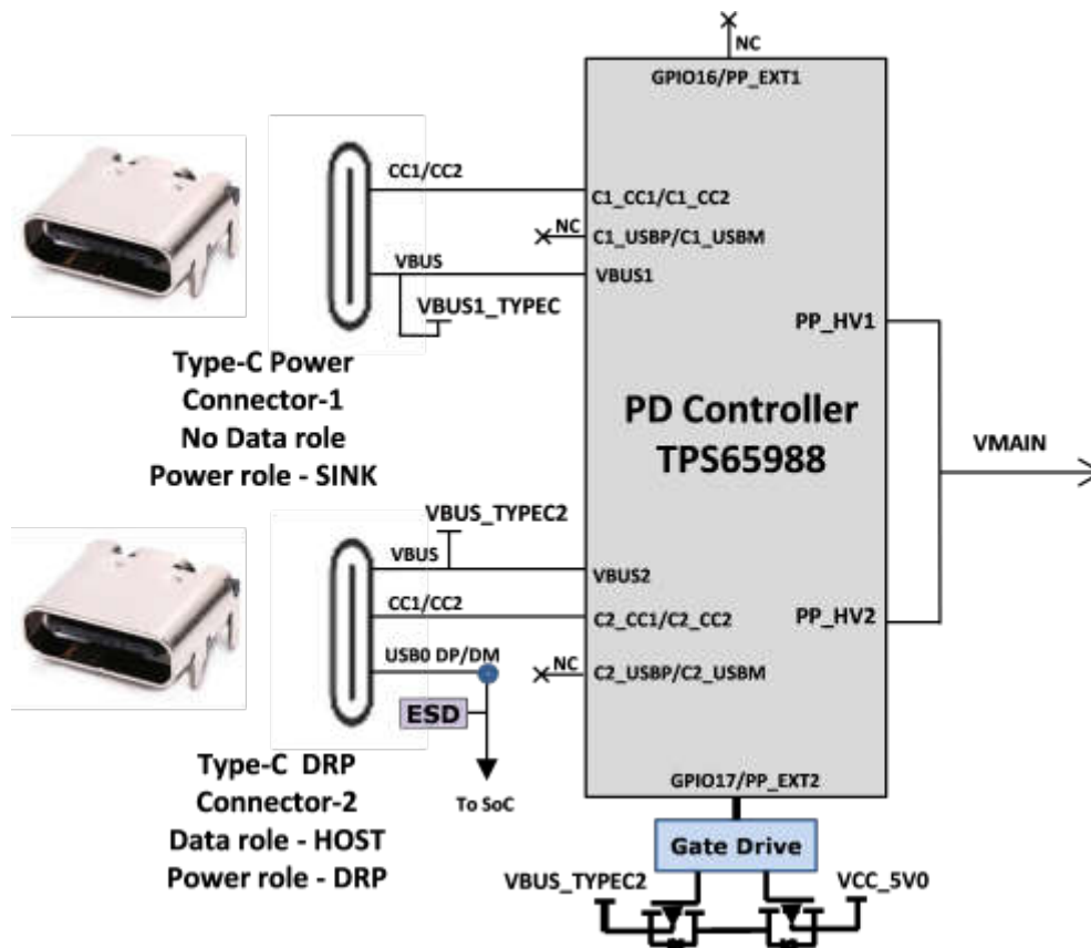
図 2-25. 電源入力
