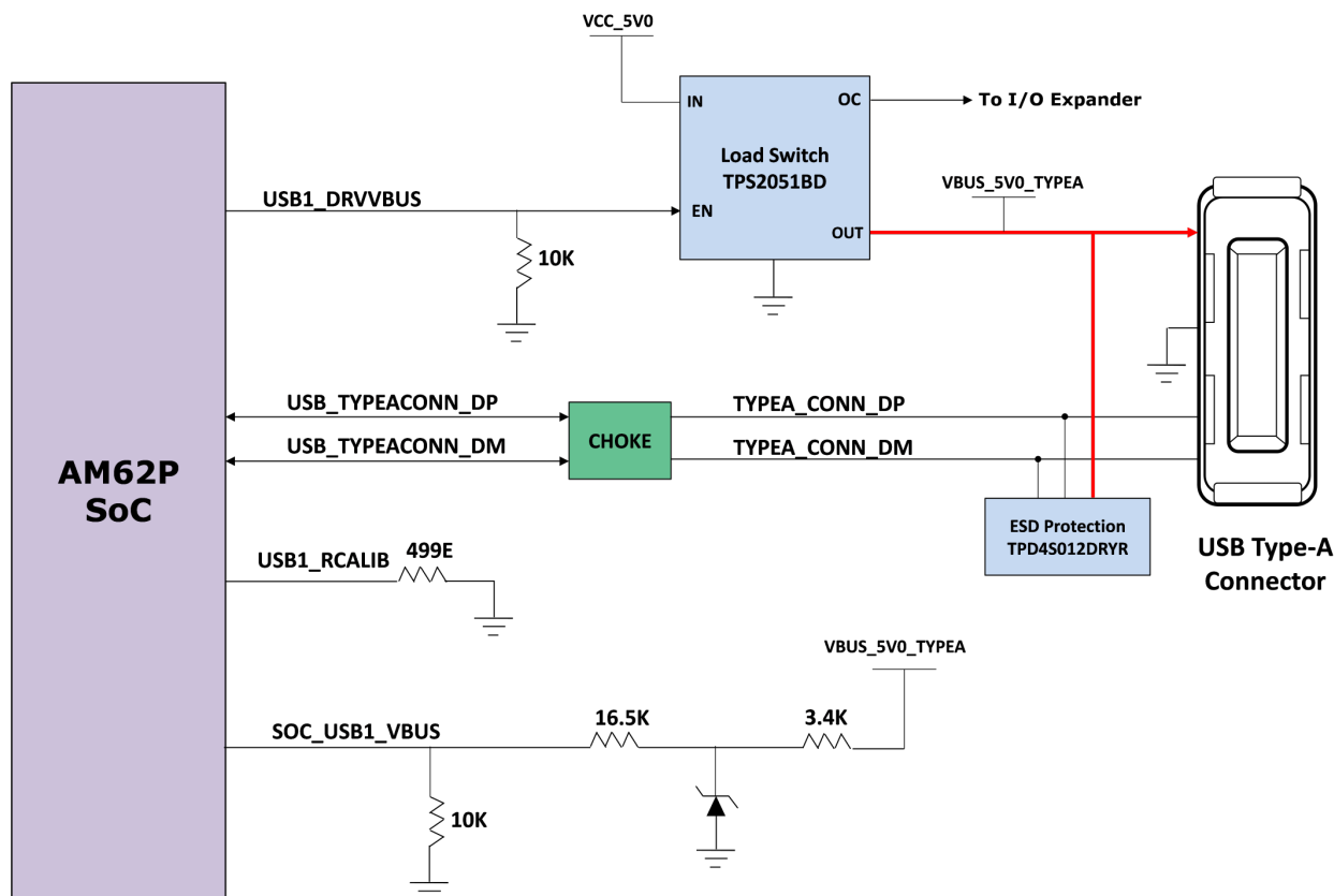
図 2-16. USB 2.0 タイプ A インターフェイス
