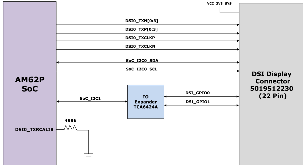
図 2-10. DSI
