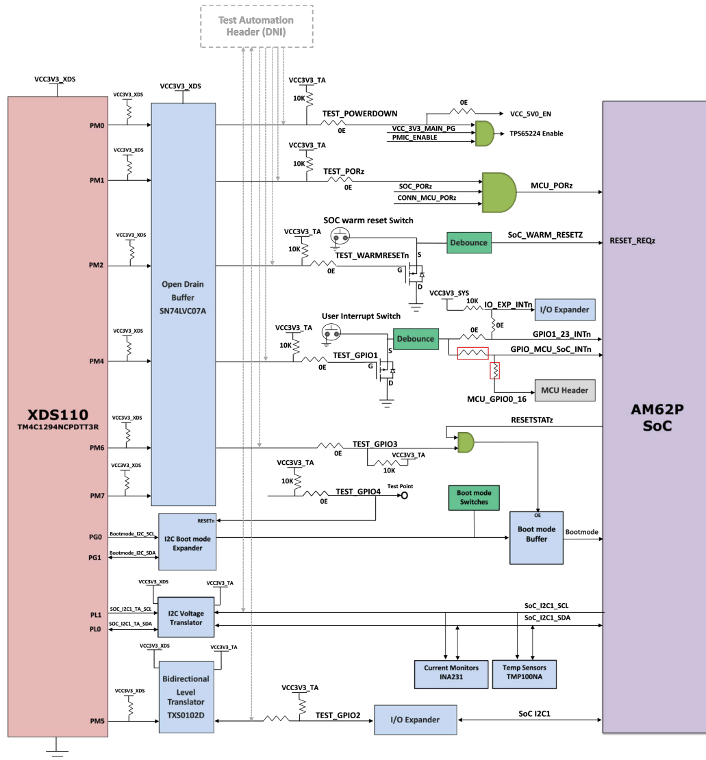
図 2-14. テスト オートメーション インターフェイス
