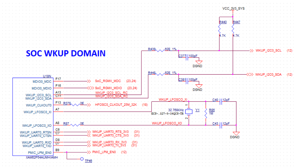
図 2-6. SOC WKUP ドメイン クロック
