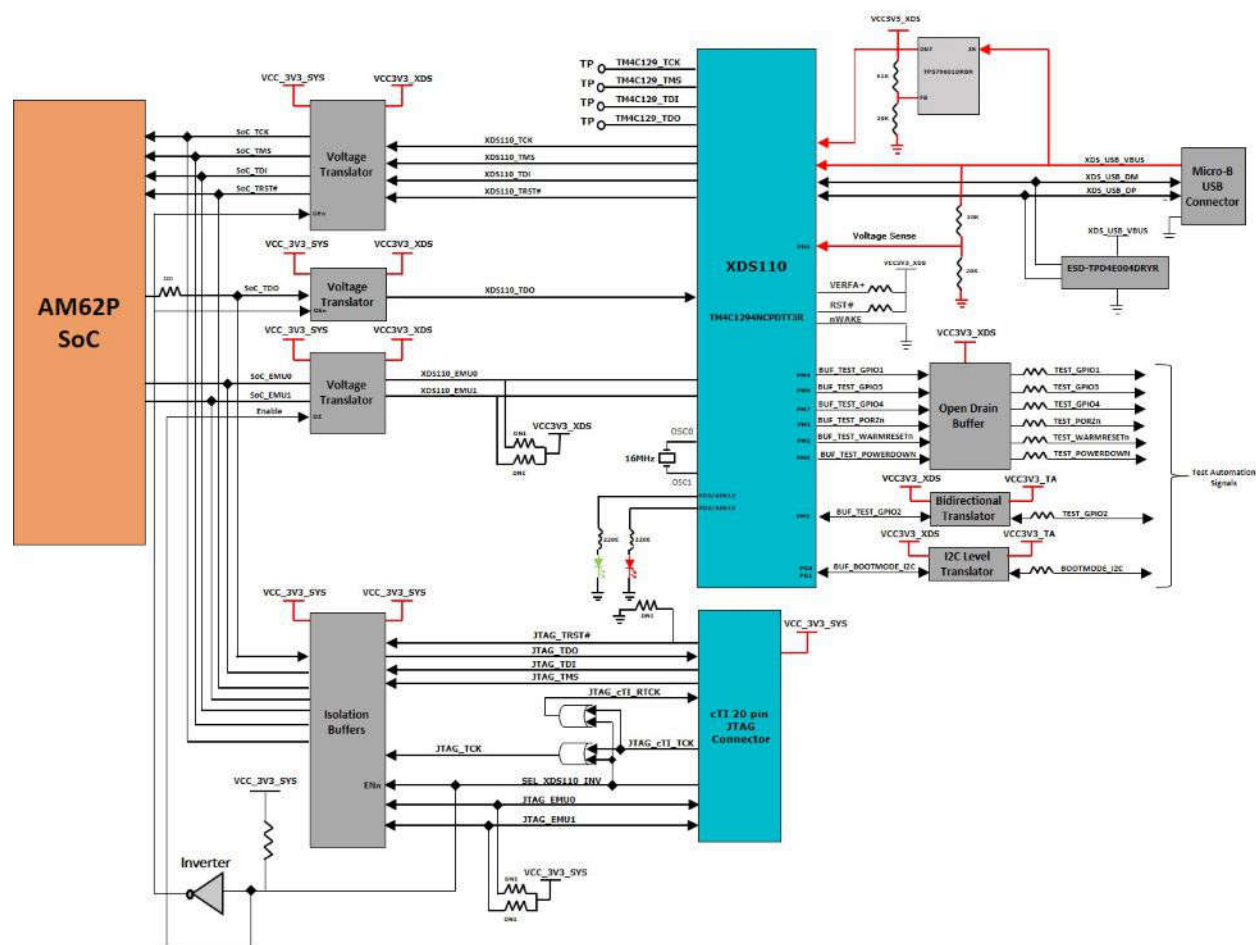
図 2-13. JTAG インターフェイス
