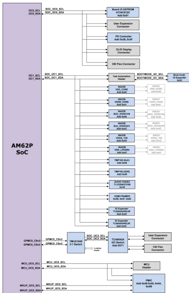
図 2-30. I2C インターフェイス
