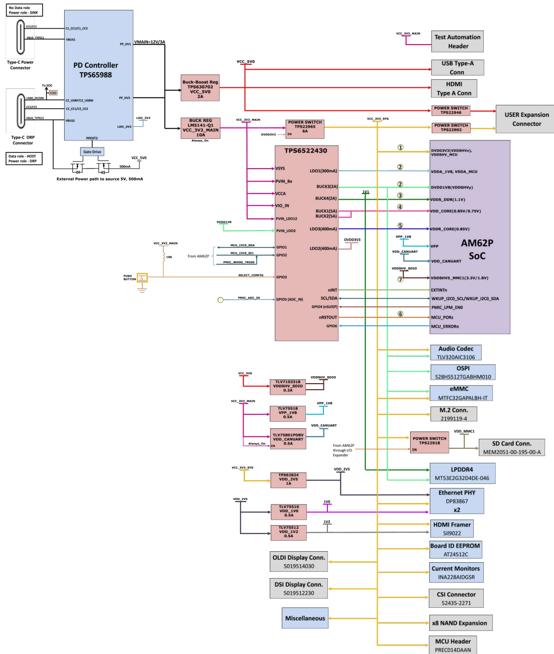
図 2-26. 電力アーキテクチャ
