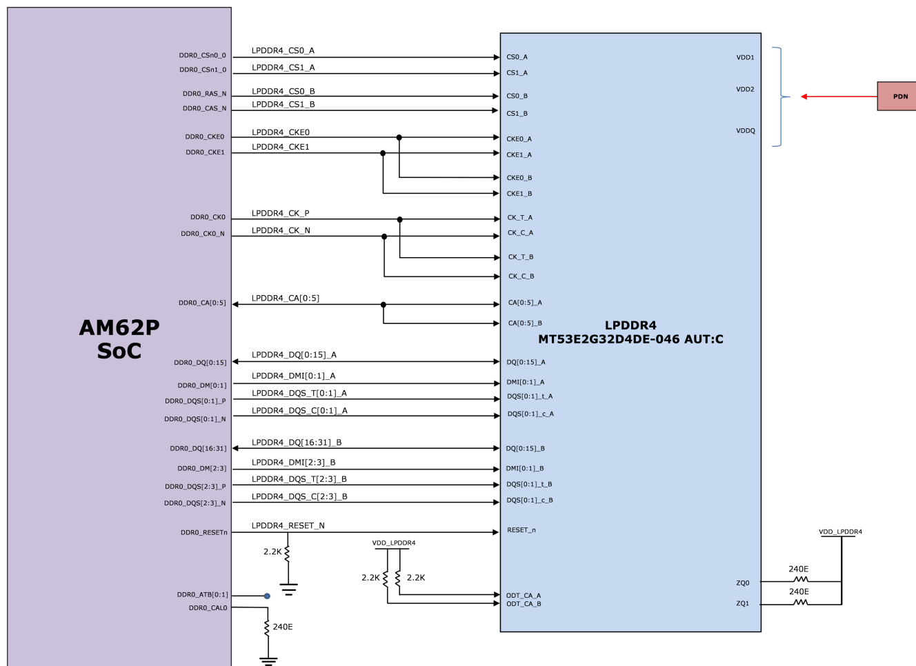
図 2-18. LPDDR4 インターフェイス
