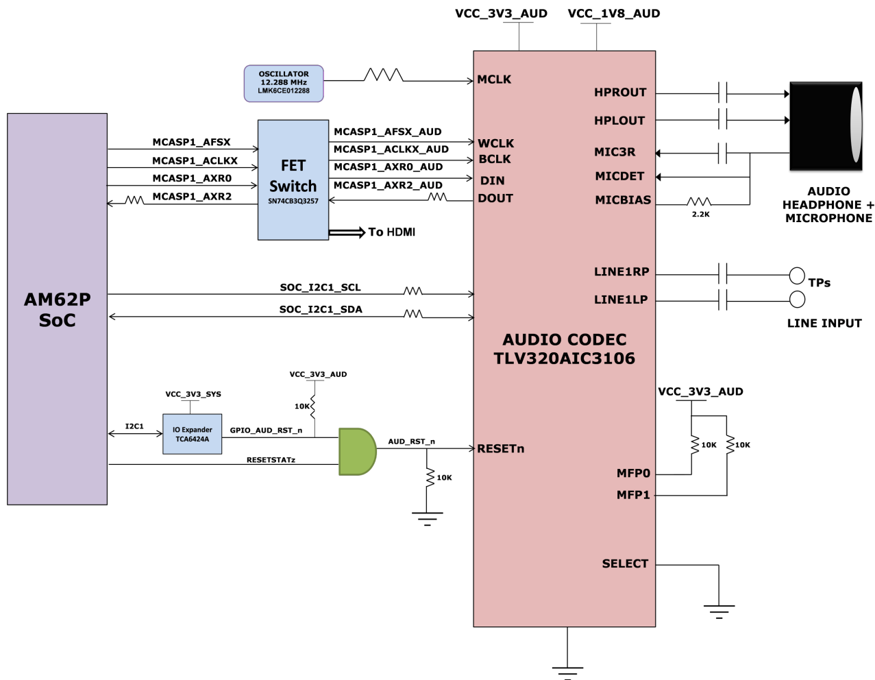
図 2-11. オーディオ コーデック インターフェイス
