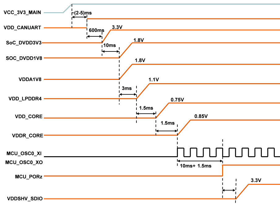
図 2-27. 電源シーケンス
