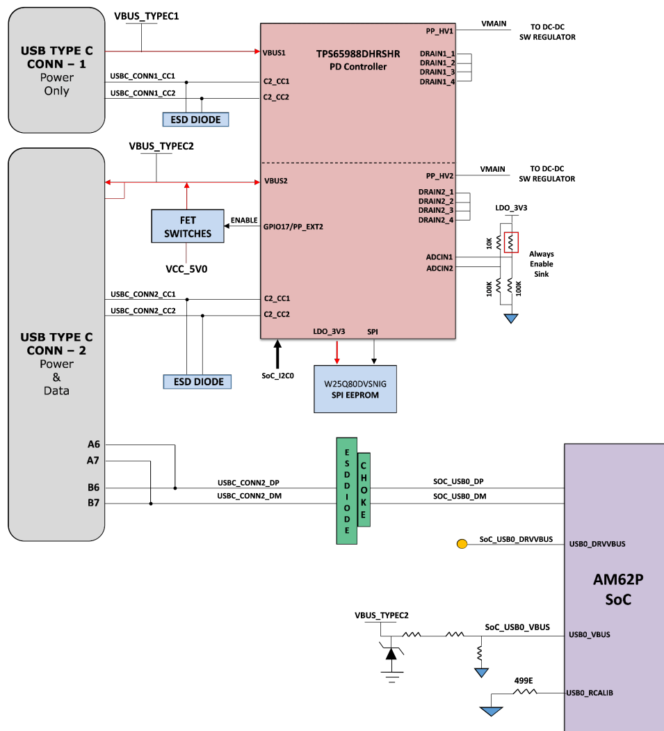
図 2-17. USB 2.0 Type C® インターフェイス
