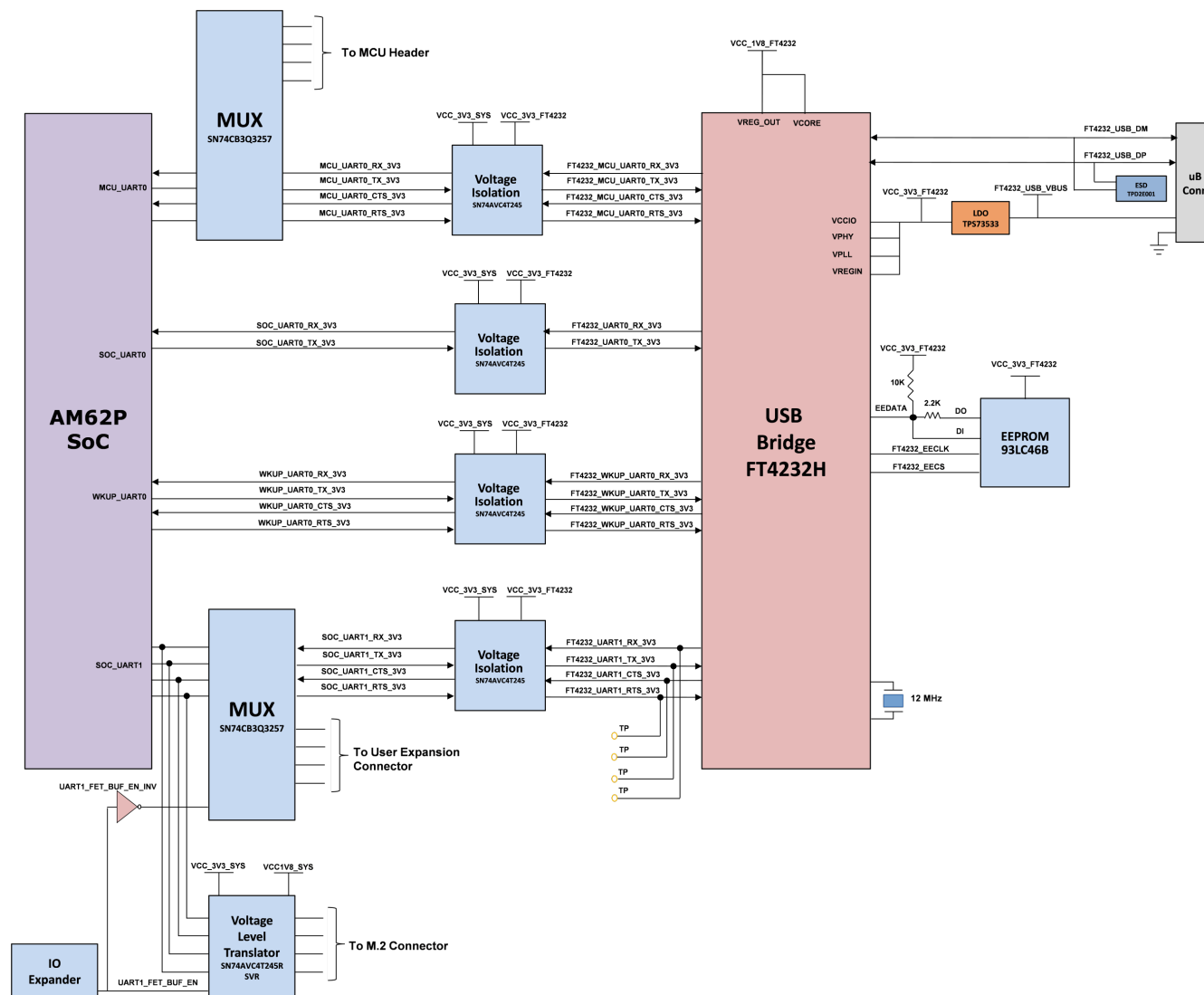
図 2-15. UART インターフェイス
