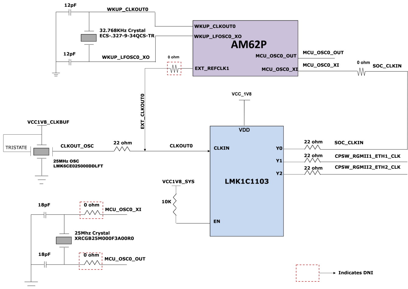
図 2-5. クロック アーキテクチャ
