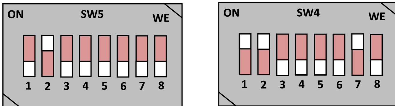
図 2-28. ブート モード スイッチ (MMCSD ブート)
