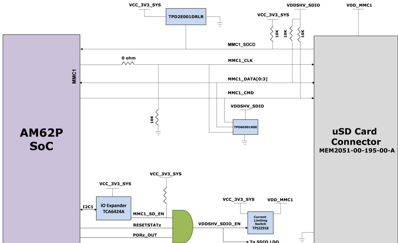
図 2-21. uSD インターフェイス
