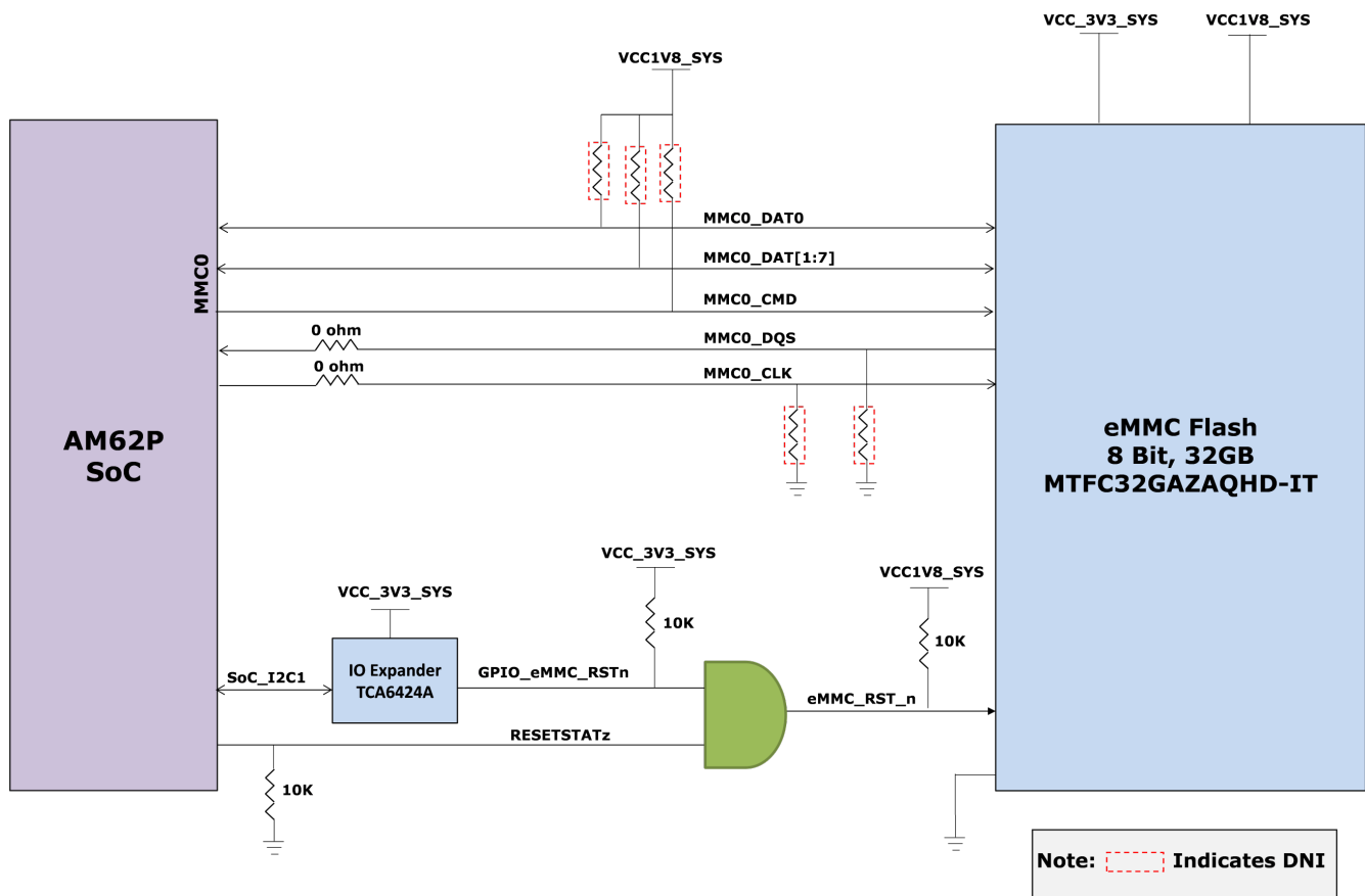
図 2-20. eMMC インターフェイス
