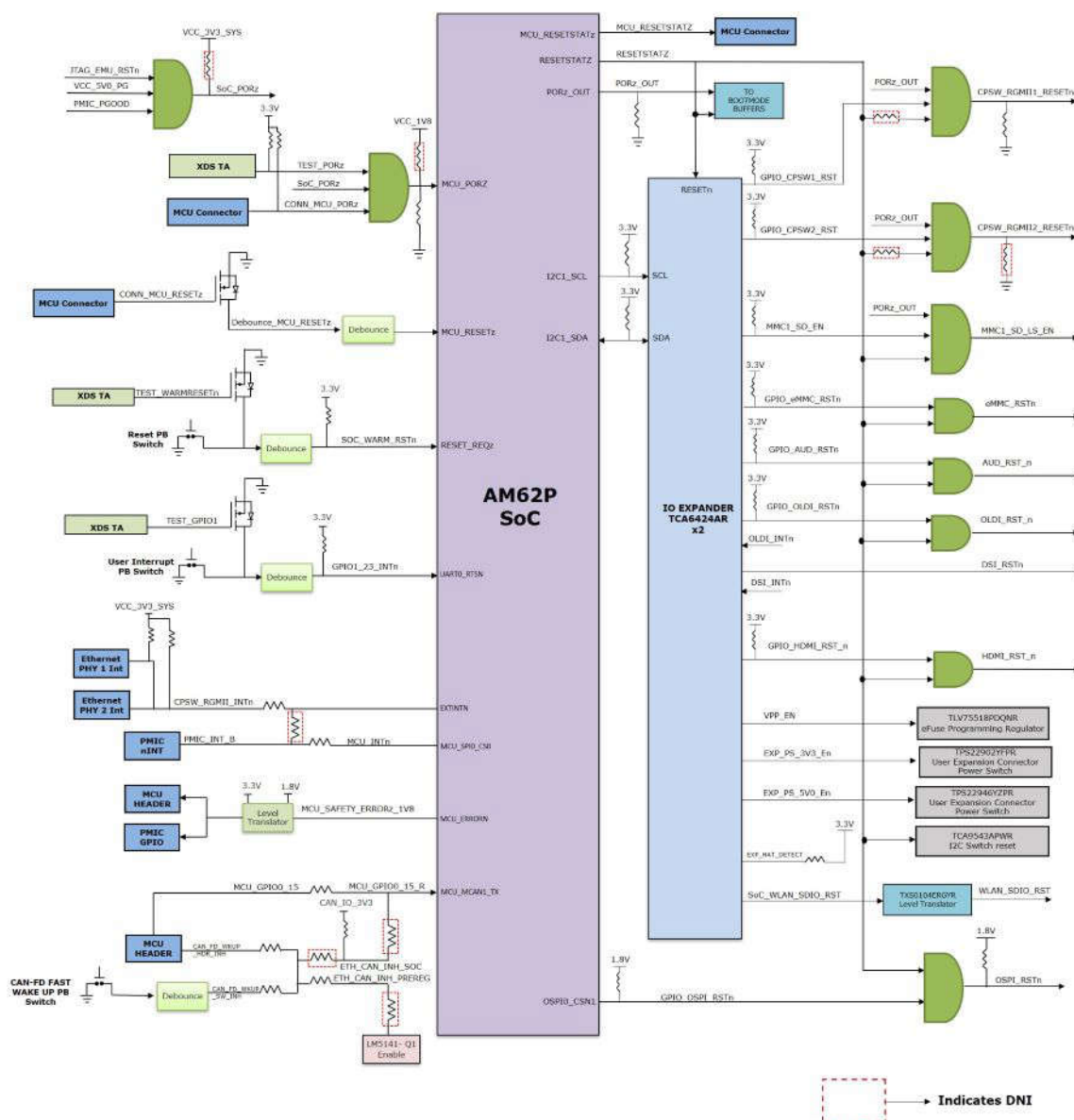
図 2-7. リセット アーキテクチャ
