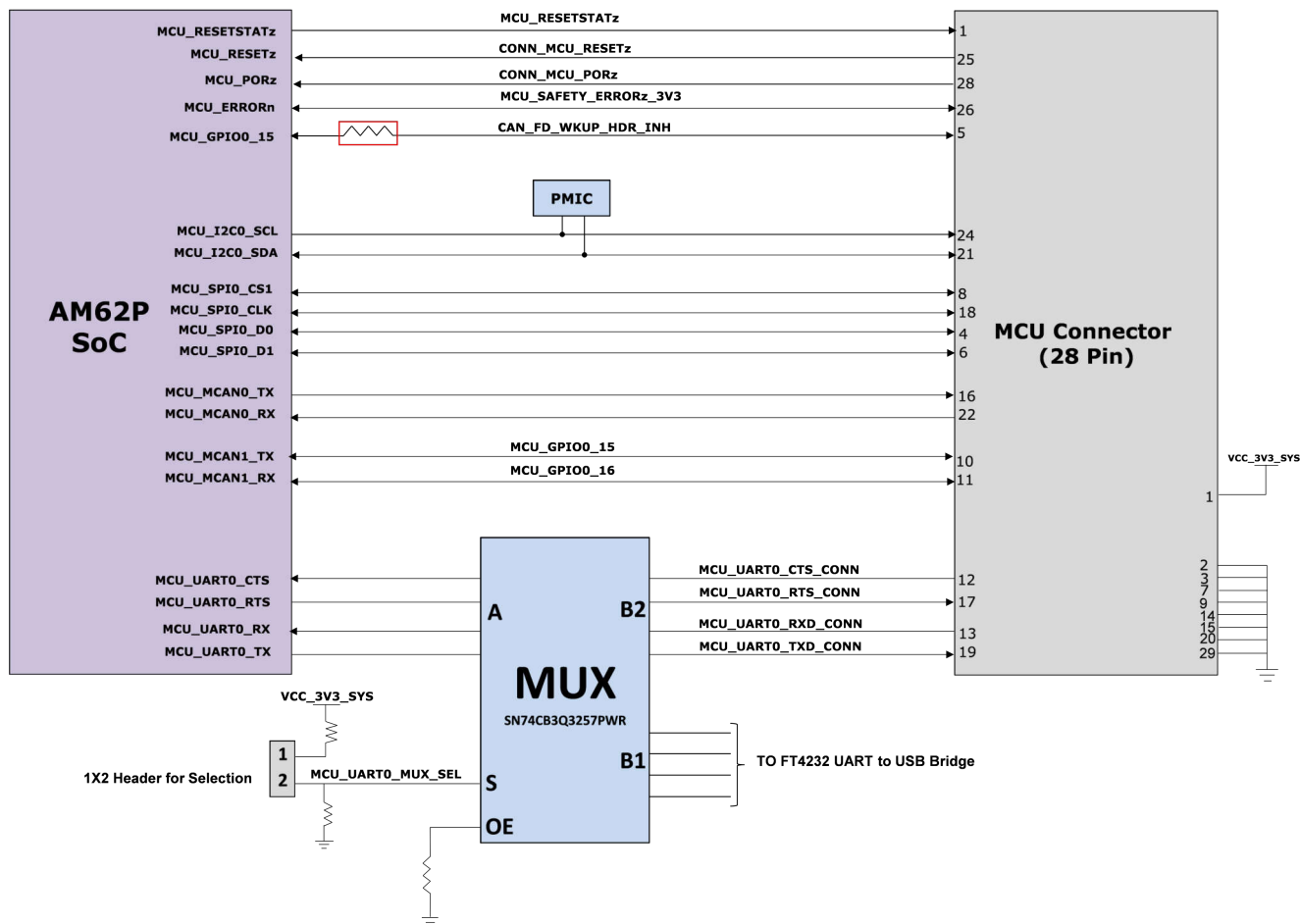
図 2-29. マイコン コネクタ インターフェイス
