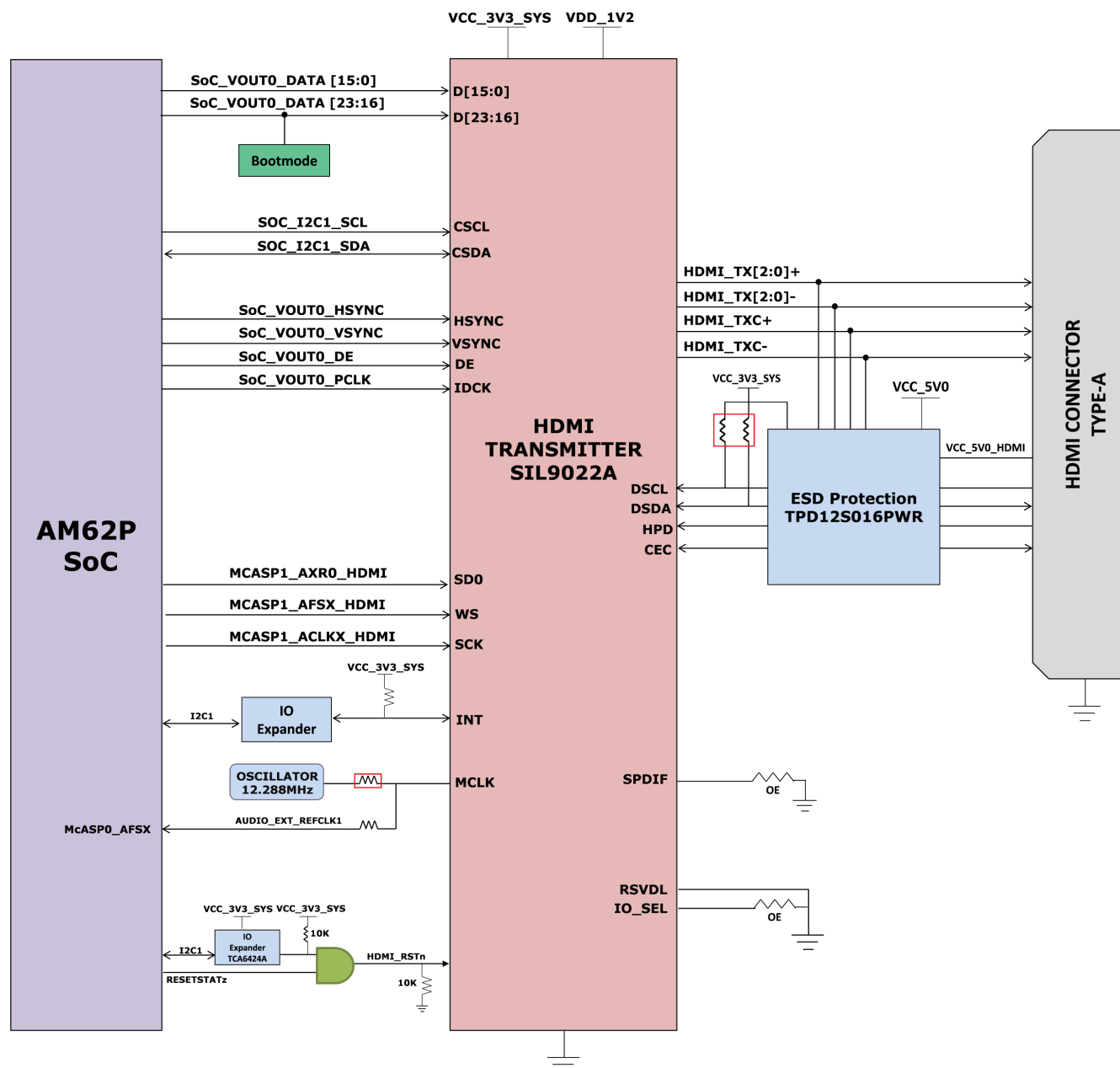
図 2-12. HDMI
