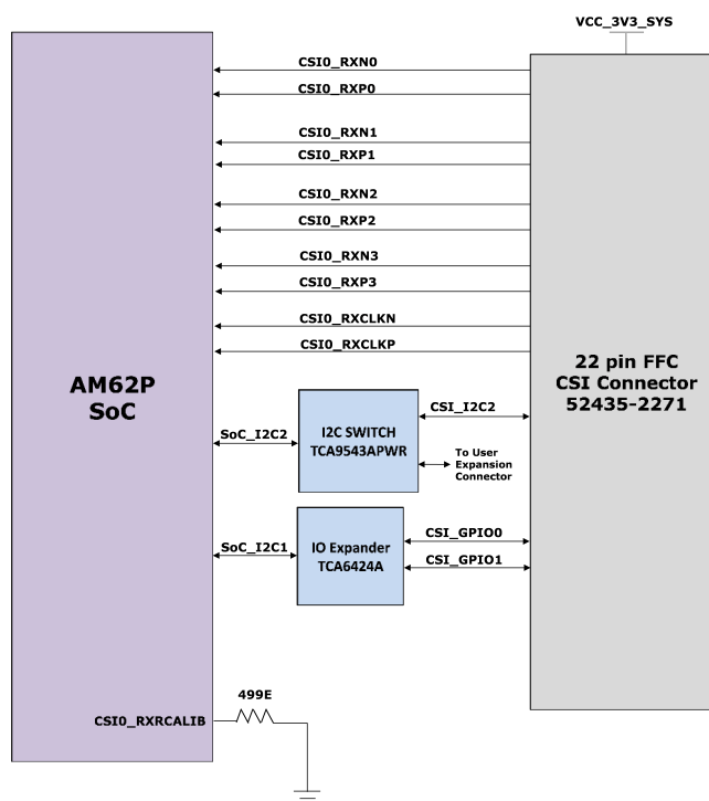
図 2-8. CSI
