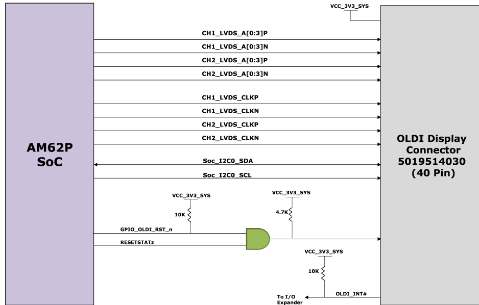
図 2-9. OLDI
