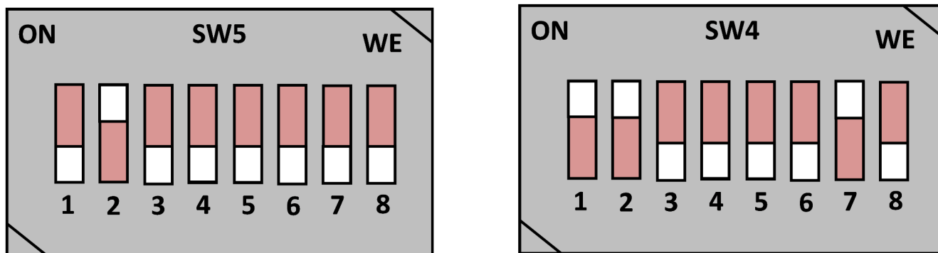
図 2-4. ブート モードの例 (MMCSD ブート)
