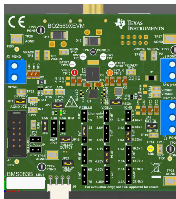
BQ25690EVM REV B ハードウェア ボード
