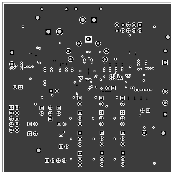
図 4-4. BMS083B 内部 1 層
