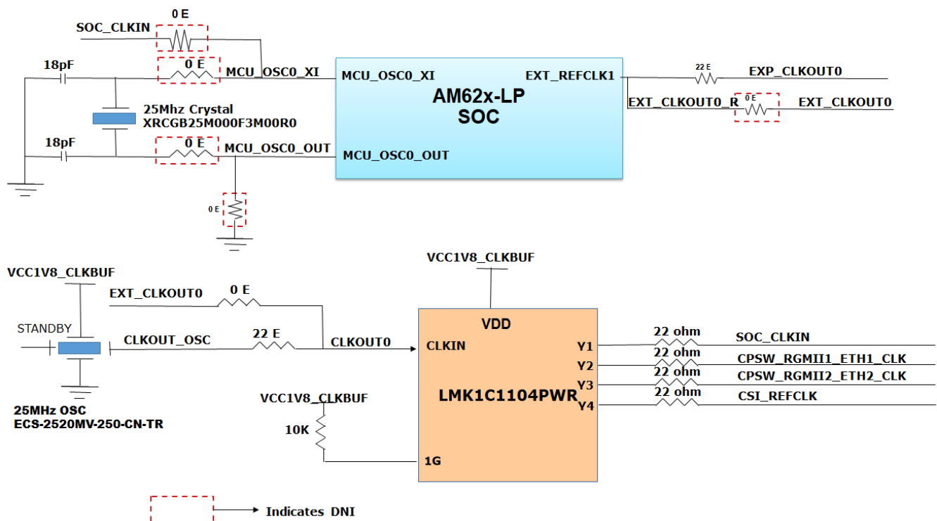
図 2-6. クロック アーキテクチャ
