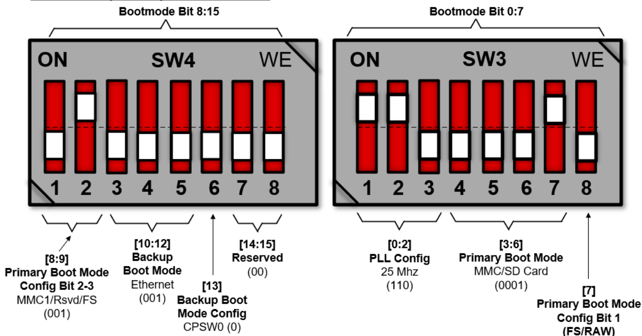
図 2-25. ブート モード切り換えの例
