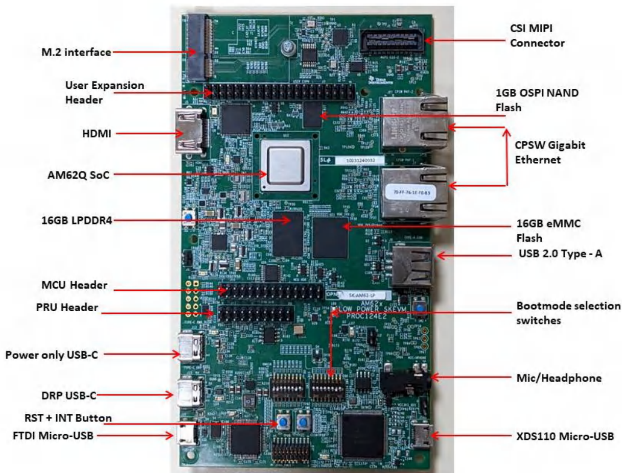
図 2-1. SK 評価基板上面
