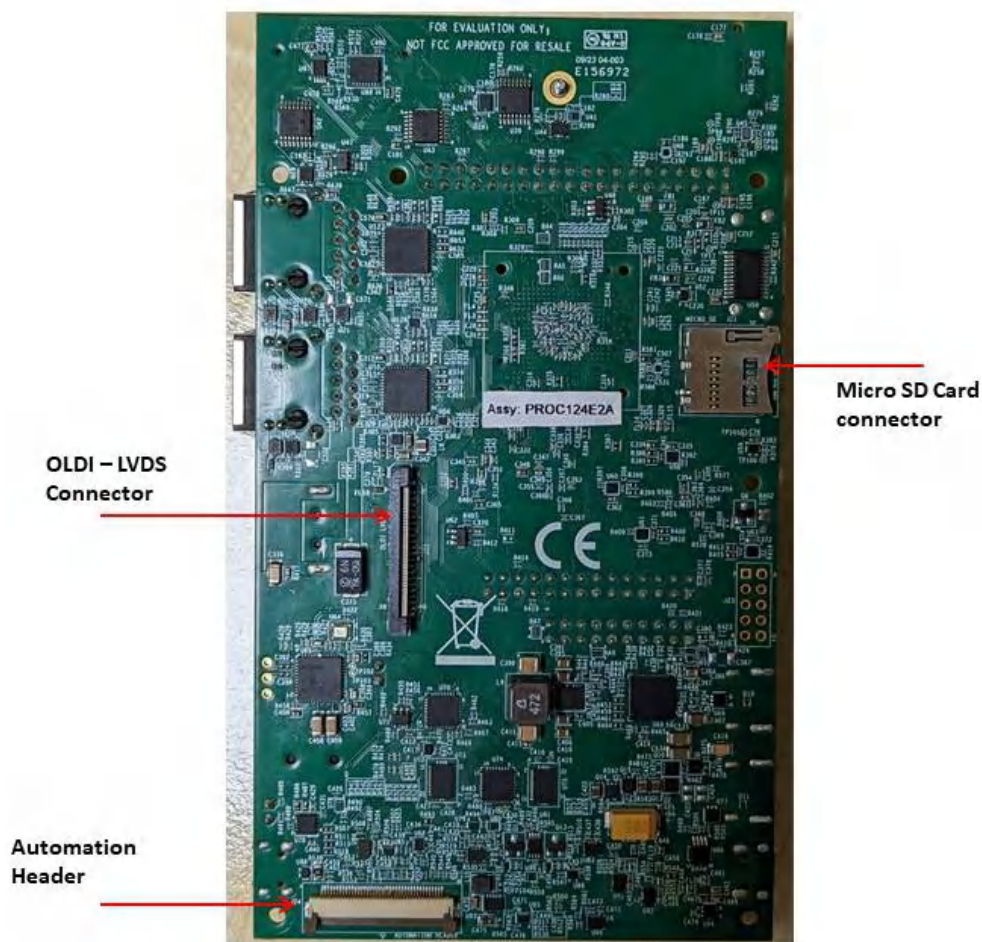
図 2-2. SK 評価基板底面
