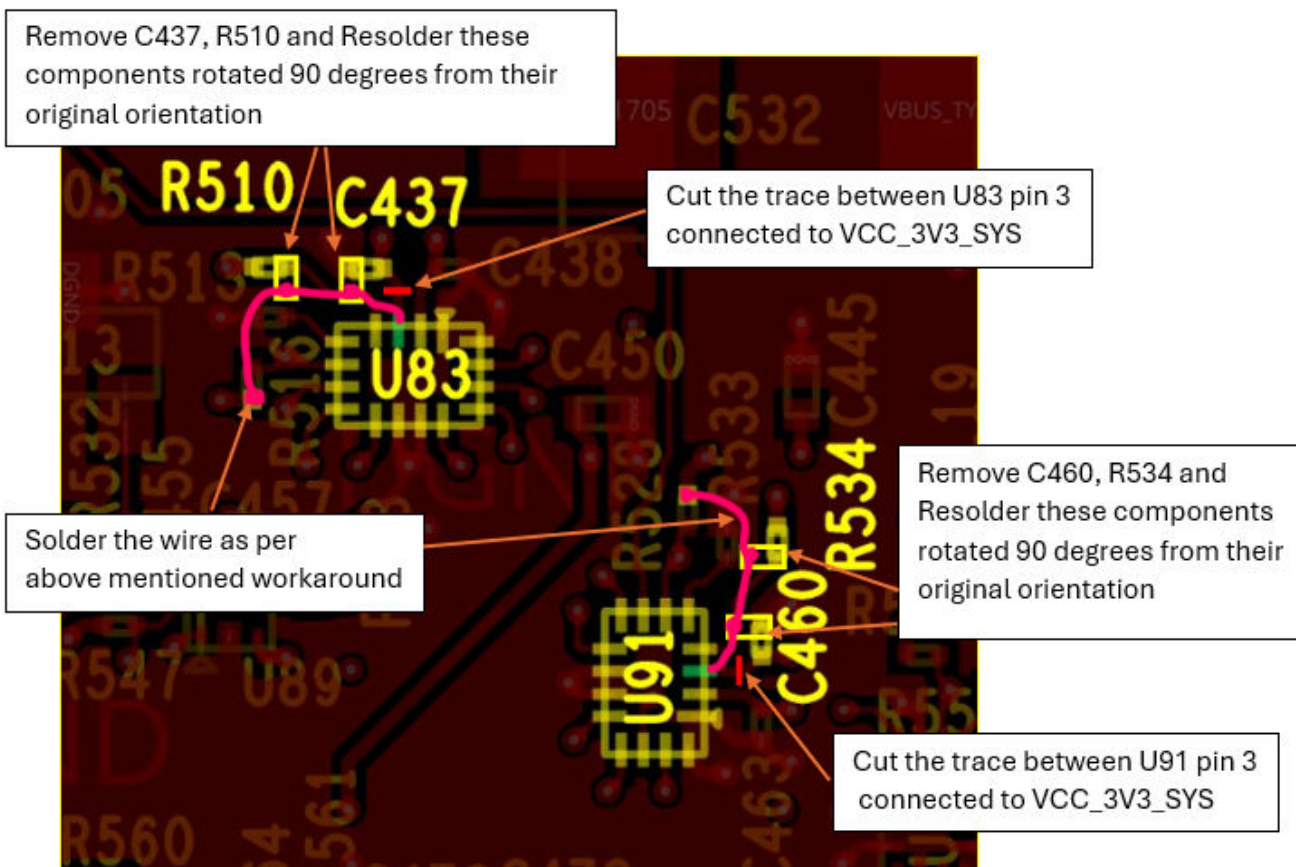
図 5-1. SK-AM62-LP 底面
