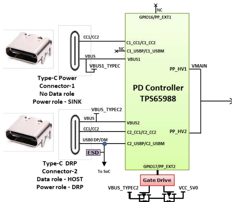
図 2-3. 電源入力ブロック図
