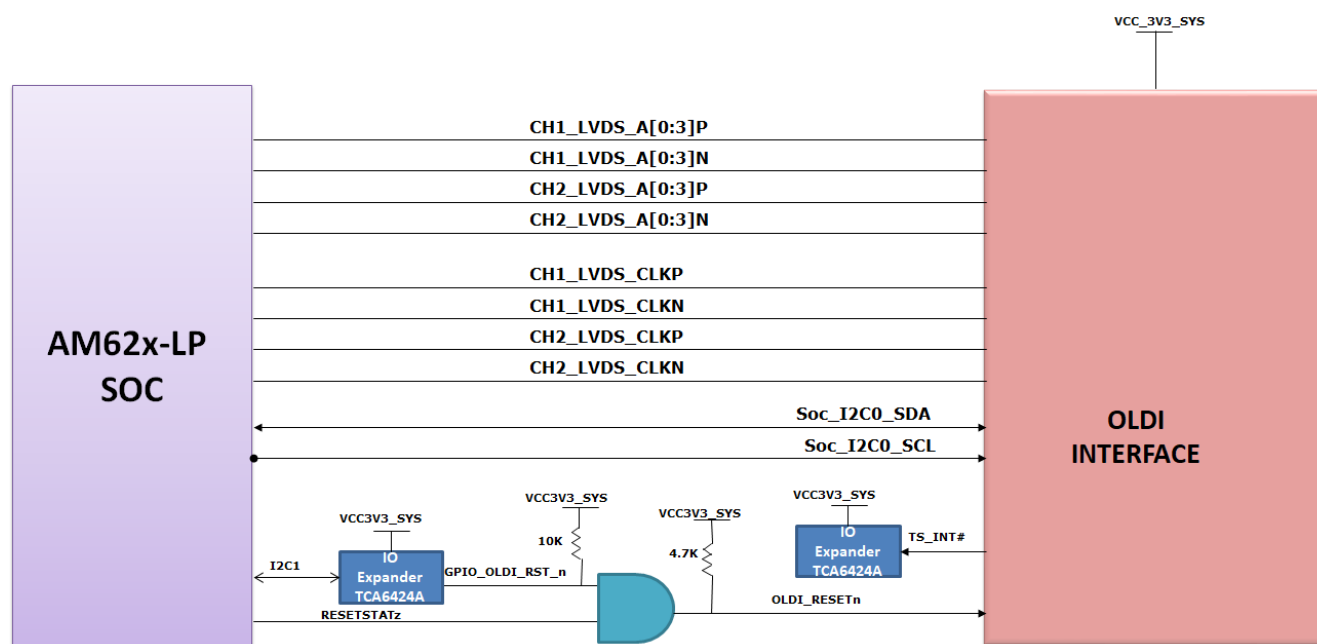
図 2-9. OLDI インターフェイスのブロック図
