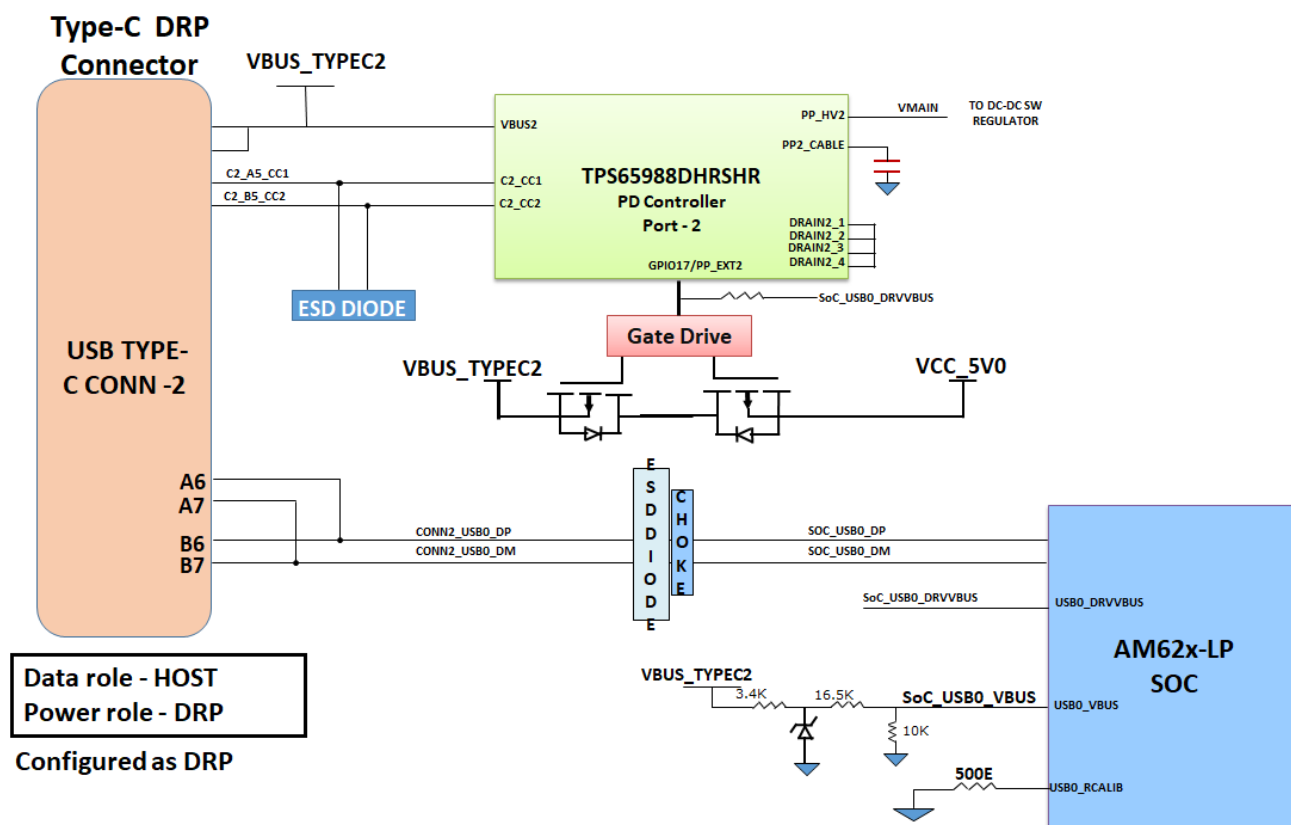
図 2-17. USB2.0 Type-C インターフェイスのブロック図
